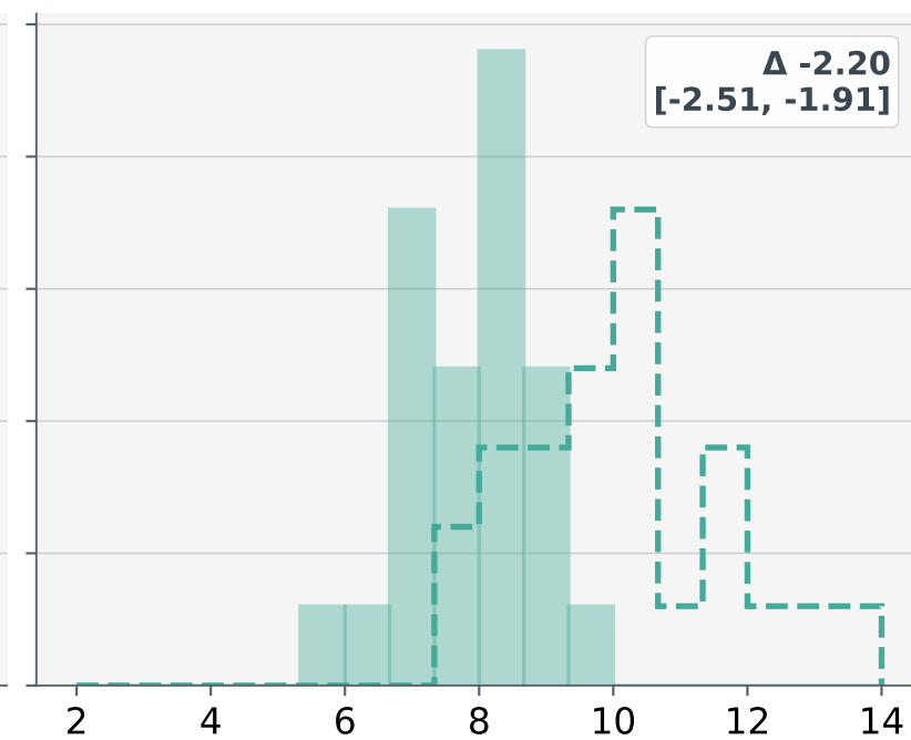
Gemma 4 31B
