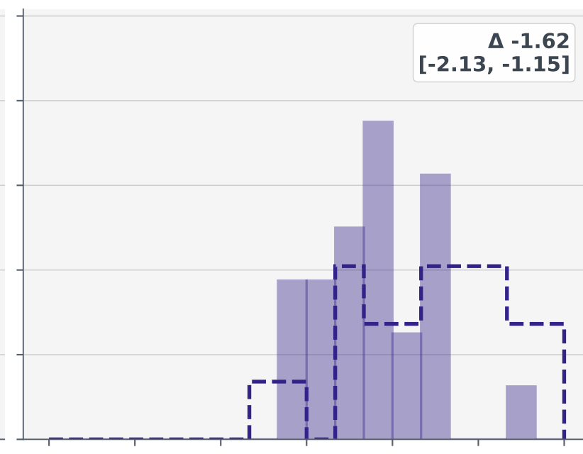
Gemma 4 31B
