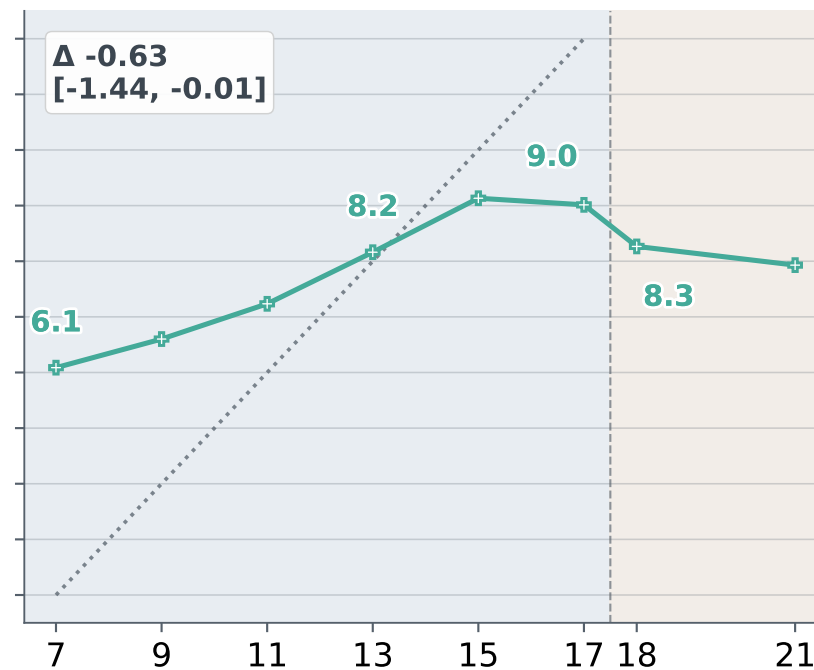
Gemma 4 31B
