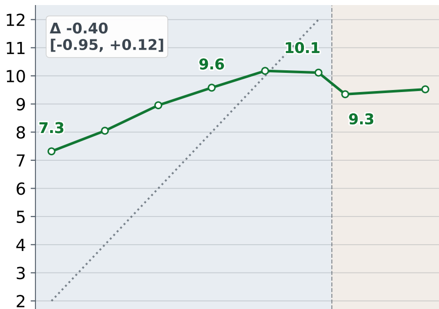
GPT-5.6 Luna
