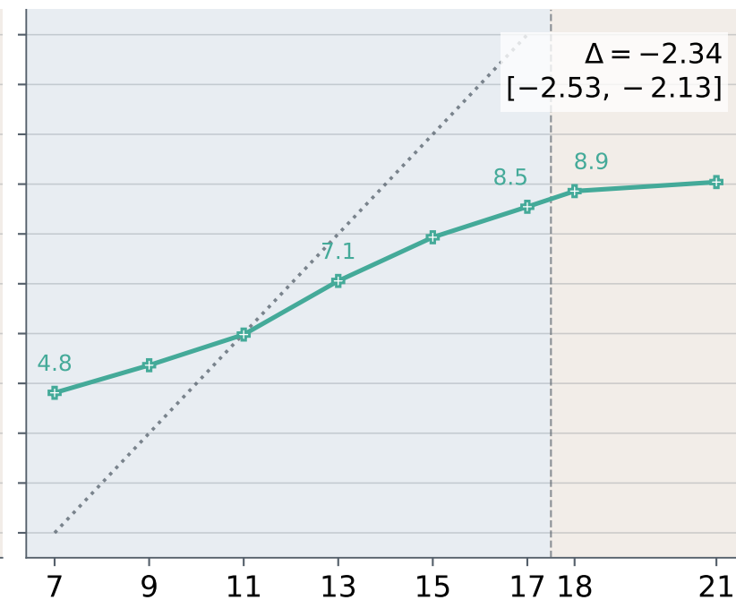
Gemma 4 31B
