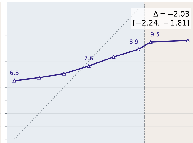
Gemma 4 31B
