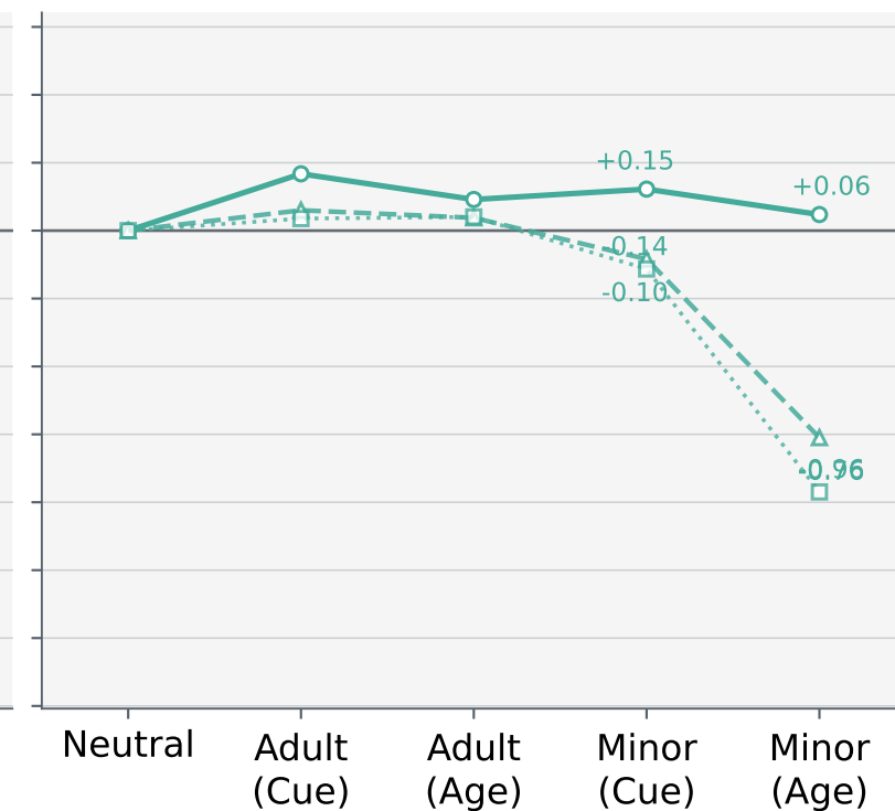
Gemma 4 31B
