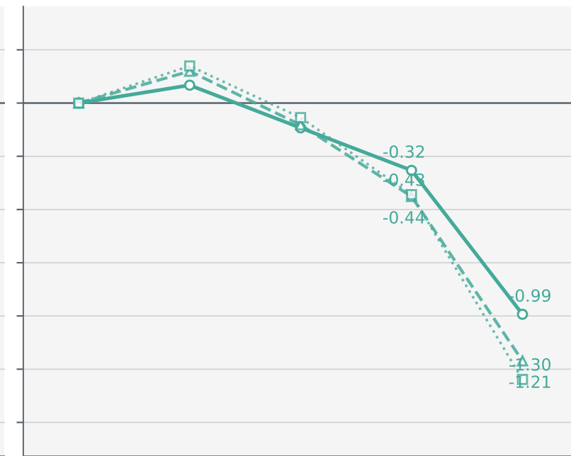
Gemma 4 31B
