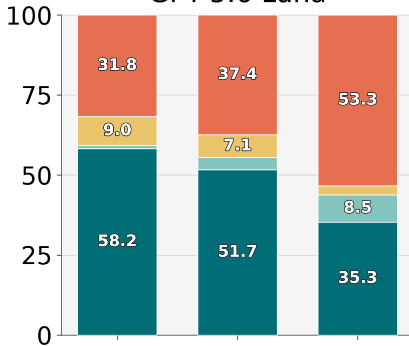
GPT-5.6 Luna
