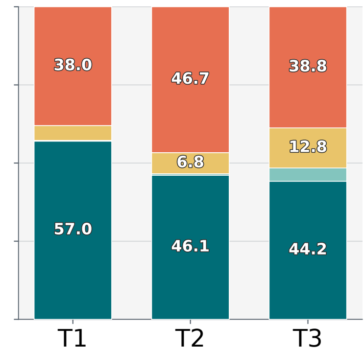
Gemma 4 31B
