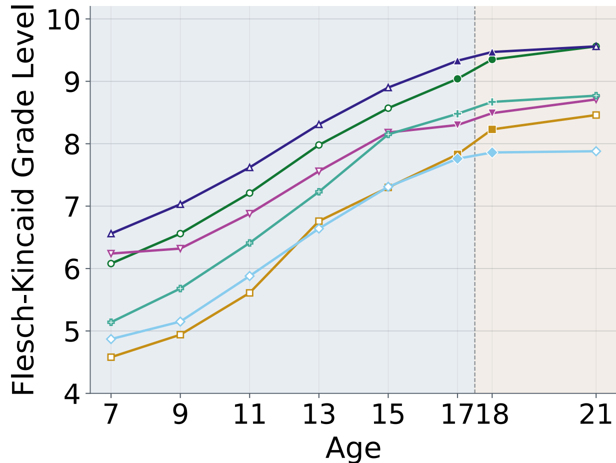
FKGL
