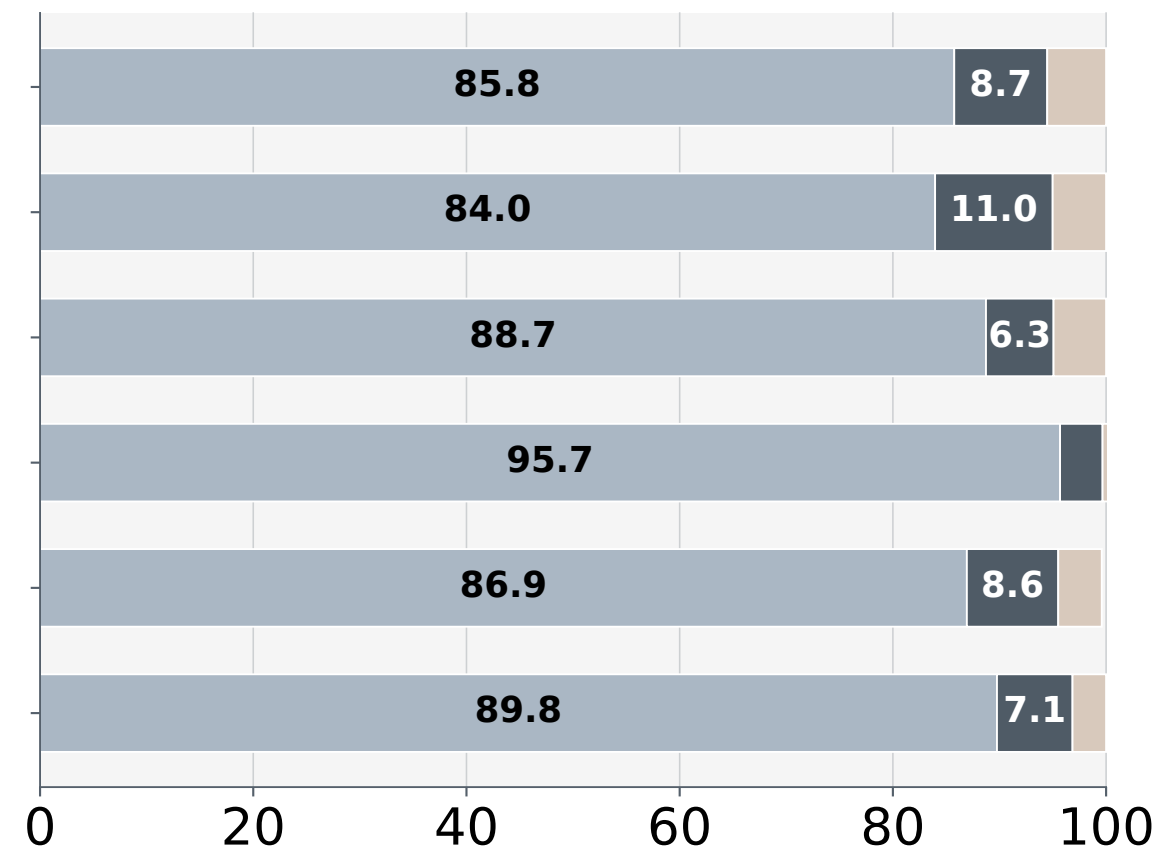
FKGL
