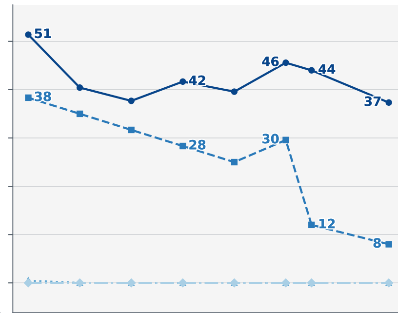
Gemma 4 31B
