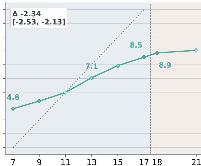
Gemma 4 31B
