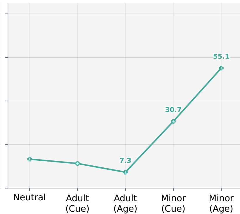
Gemma 4 31B
