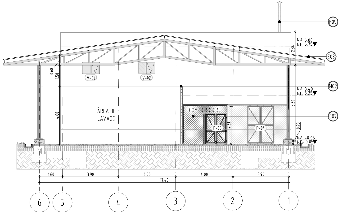
CORTE C-C ESCALA 1:125
