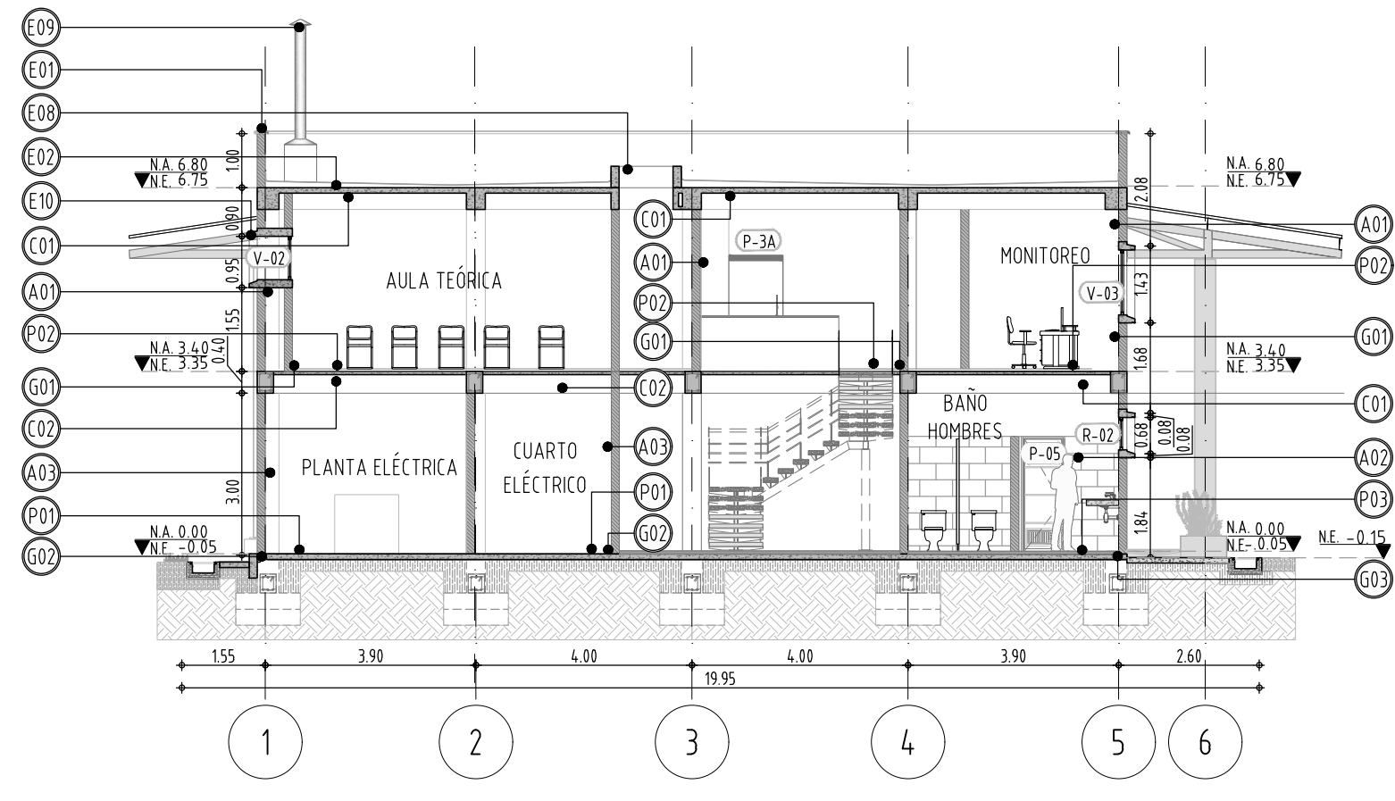
CORTE B-B ESCALA 1:125
