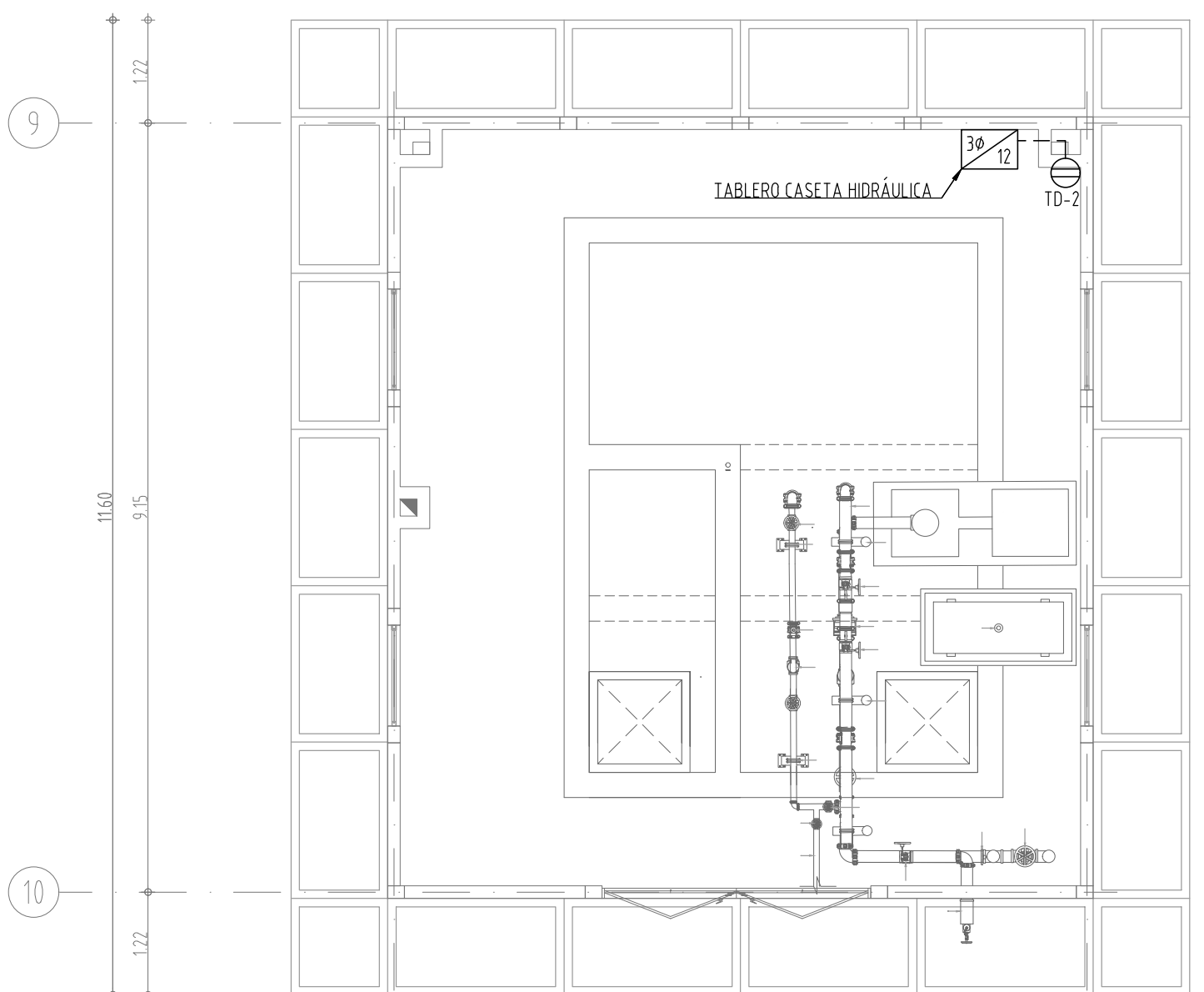
CENTRO AGUA POTABLE Y RESERVA
