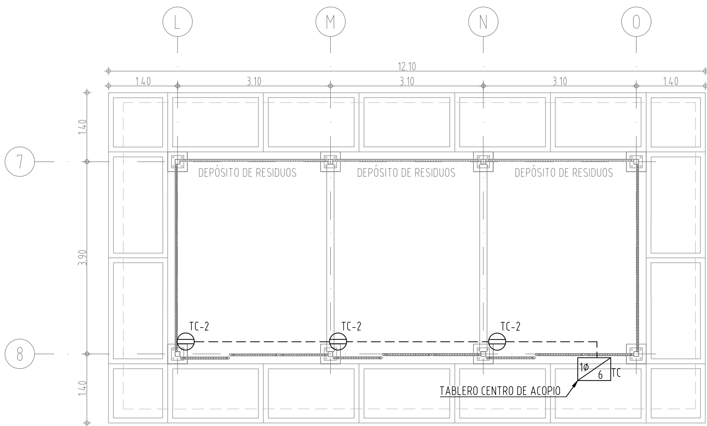
CENTRO DE ACOPIO
