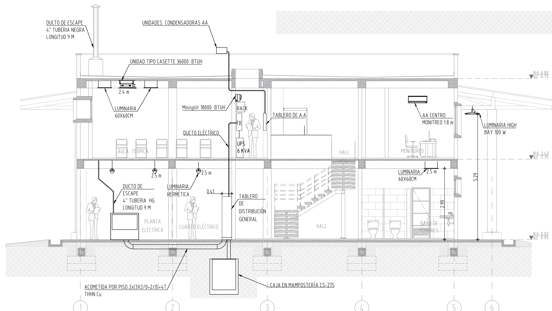
SECCIÓN 2-2 ALTURA DE INSTALACIÓN DE EQUIPOS ESCALA 1:75
