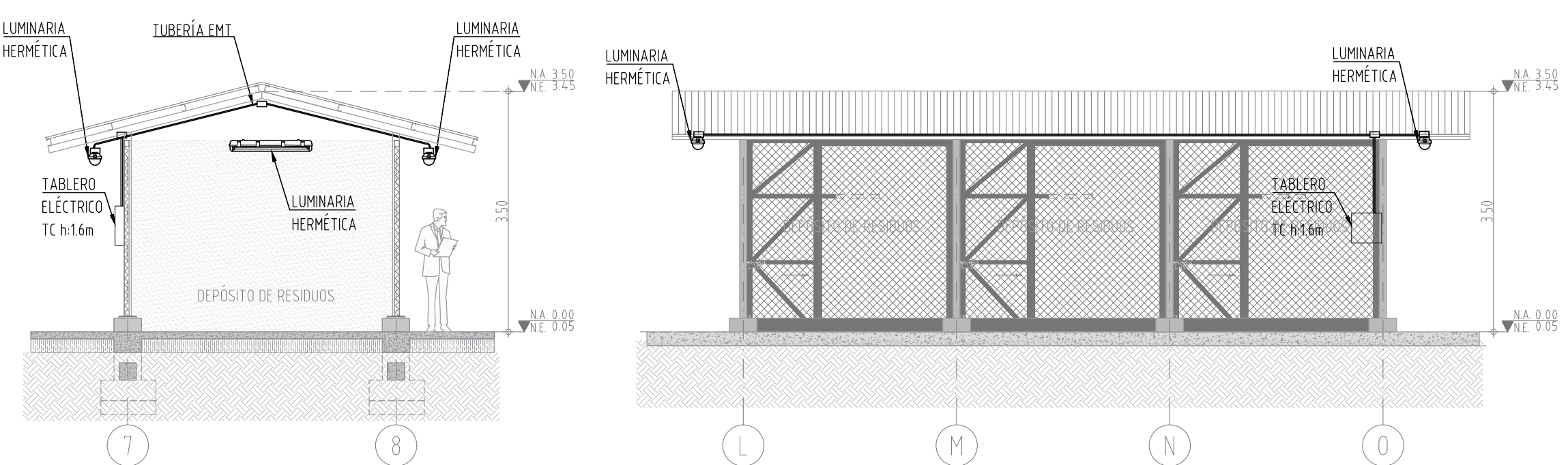
CENTRO DE ACOPIO SECCIÓN 1-1 ESCALA 1:75
