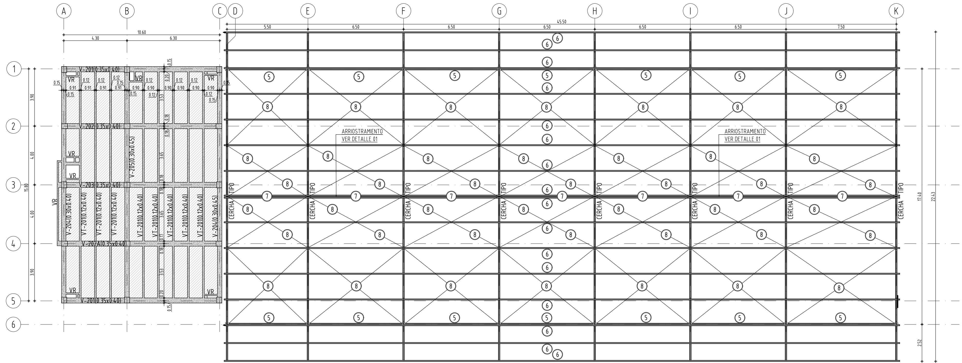
PLANTA DE CUBIERTA BLOQUE DE SERVICIO Y HANGAR ESC:1/125
