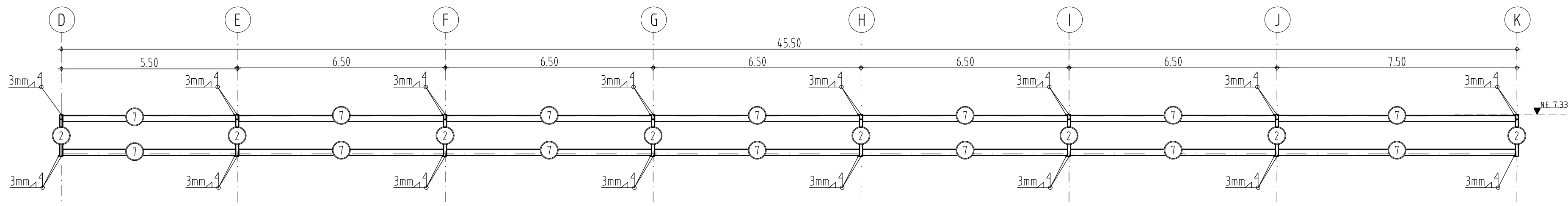
DETALLE 1 CORTE ARRIOSTRAMIENTO CERCHA (CENTRO) ESC:1/100
