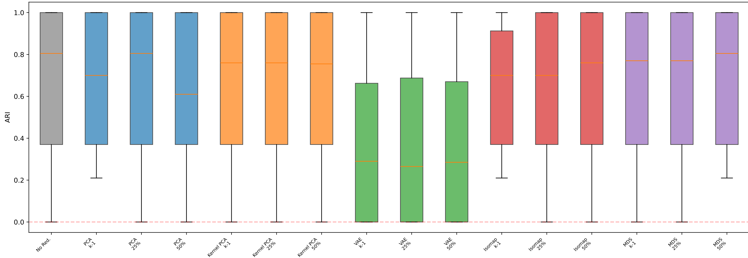
OPTICS — RSG
