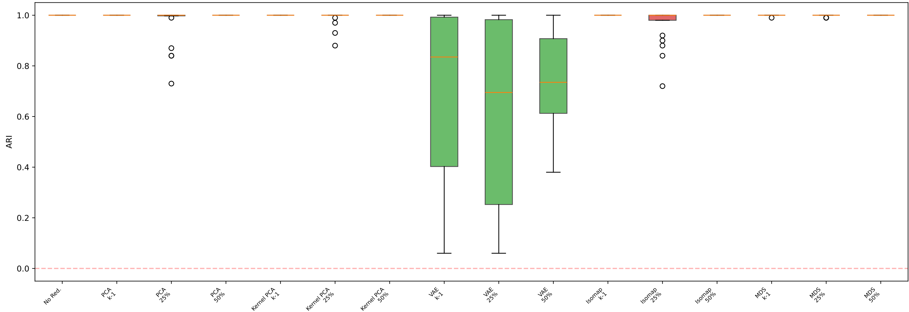
k-means — RSG
