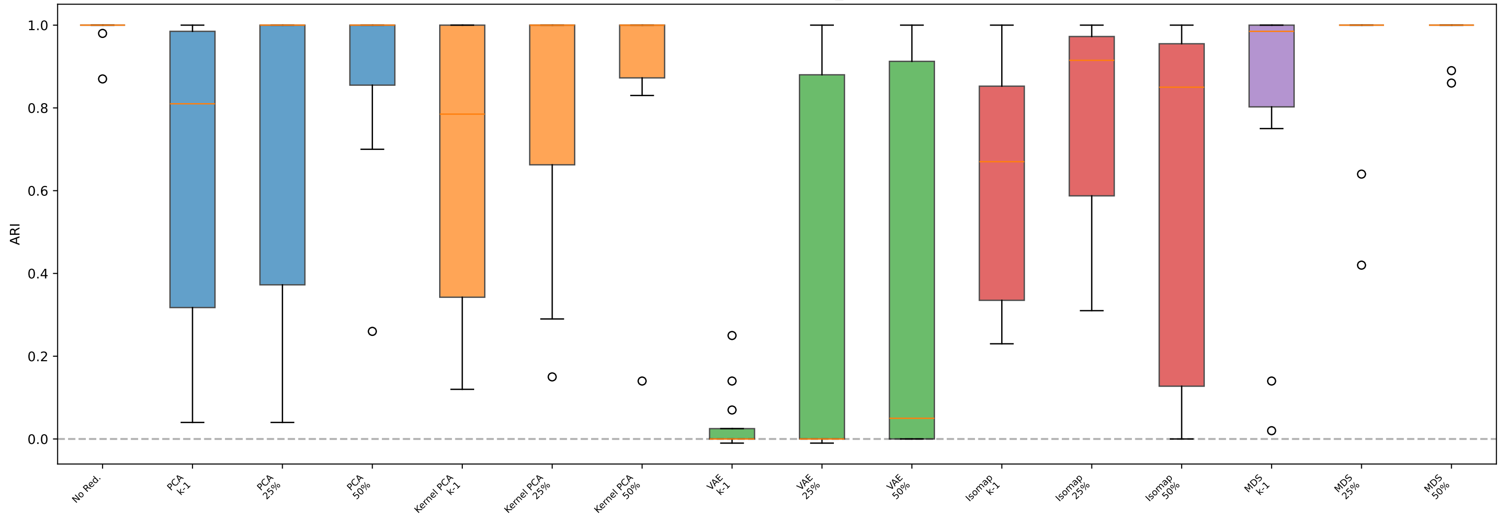
OPTICS — Synthetic_RSG
