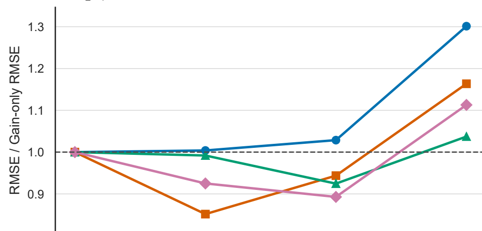
A H 2 S, Horizon 1
