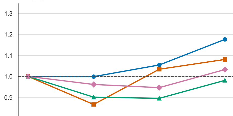
B H 2 S, Horizon 18
