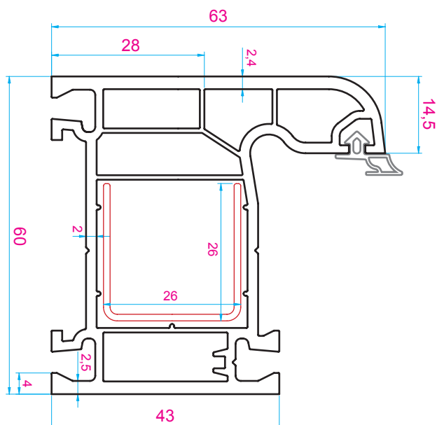
6040A-10 - 1.024 gr/m / Profil Toc - Frame Profile
