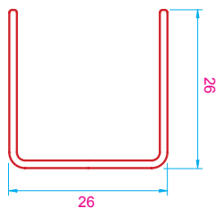
Profil Toc - Profil Aripa - Profil Teu Frame, Sash, Mullion
