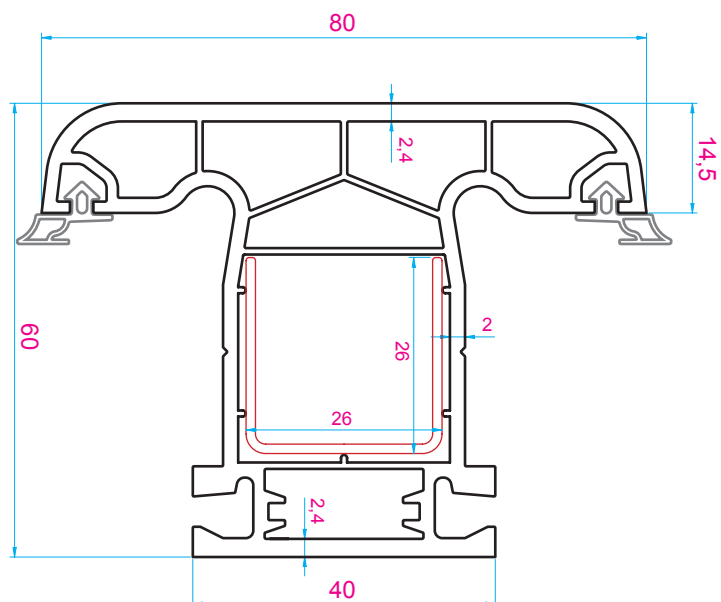
6040A-30 - 1.151 gr/m / Profil Teu - Mullion Profile
