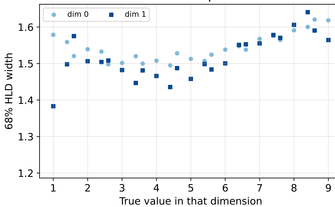
uniform: HLD width per dimension
