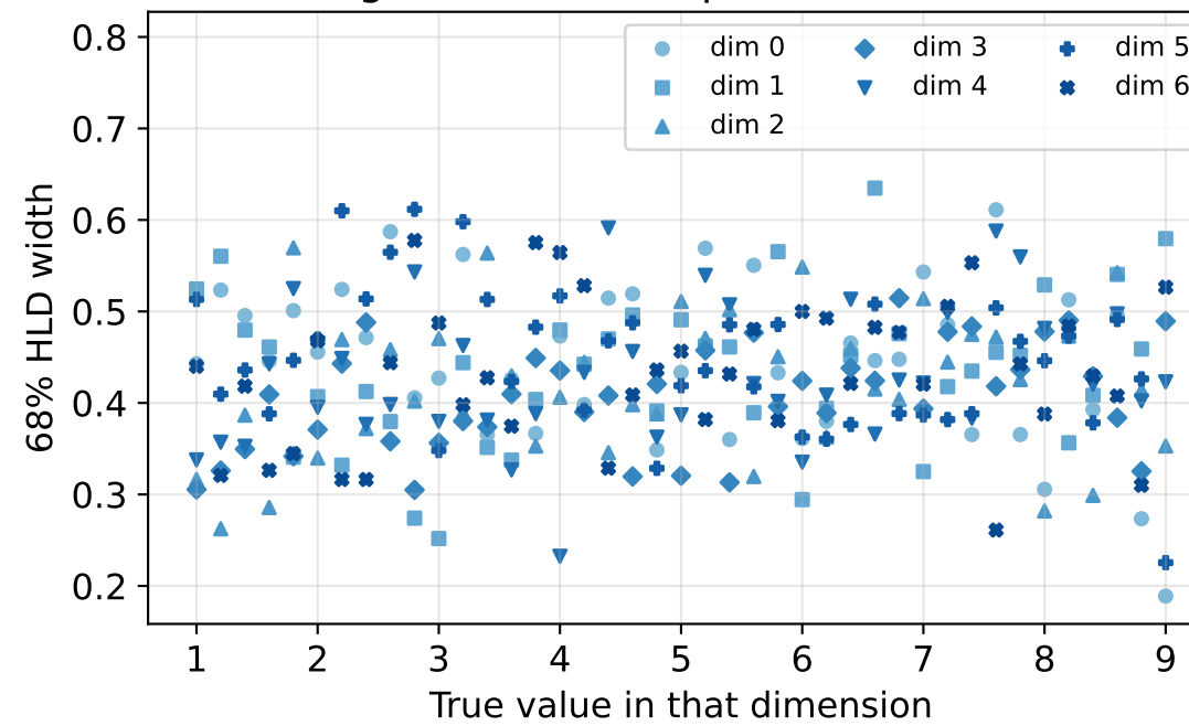
grid: HLD width per dimension
