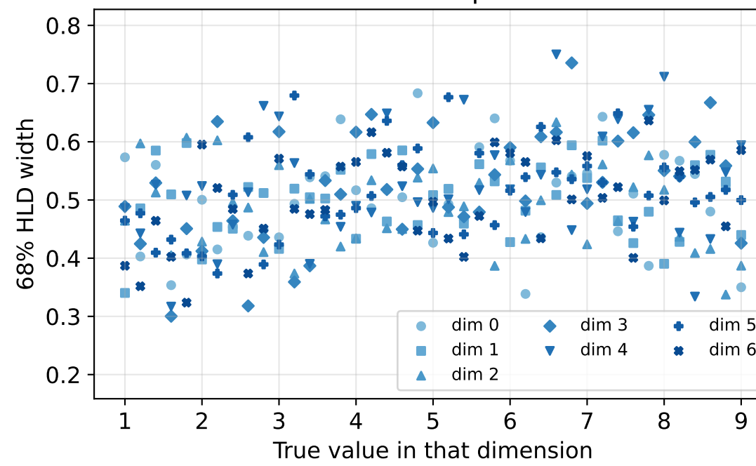
normal: HLD width per dimension
