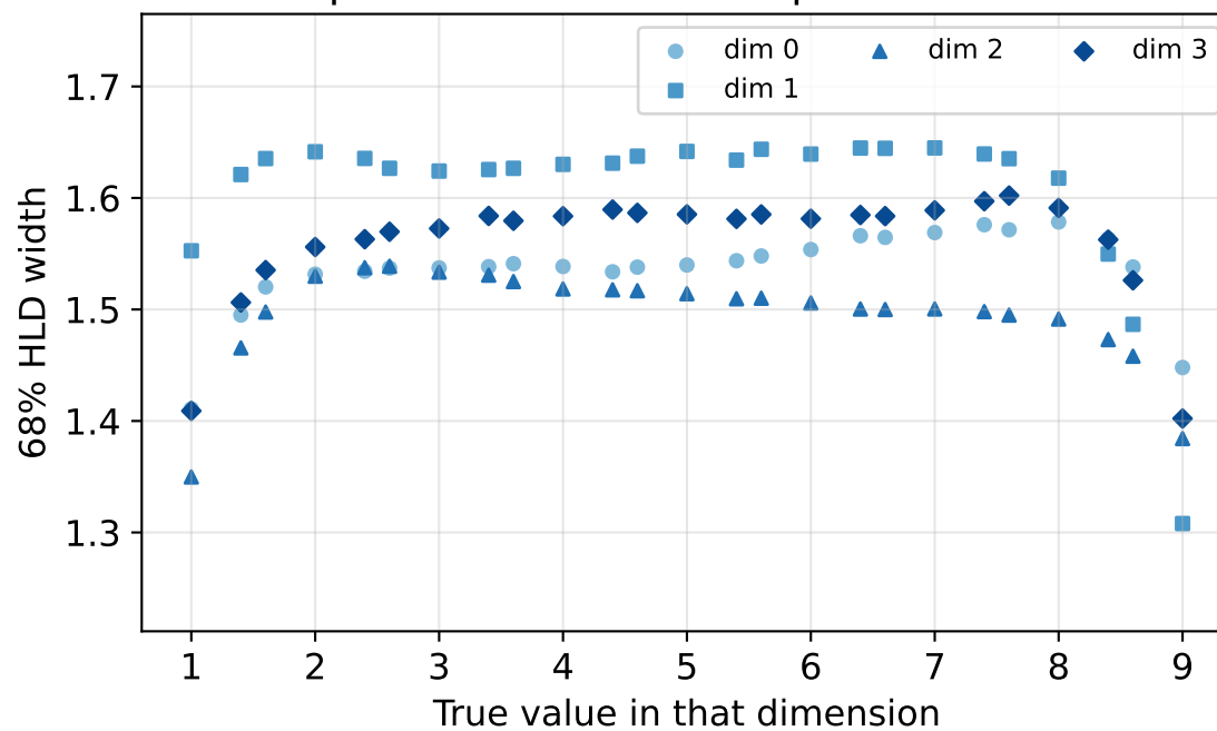
uniform: HLD width per dimension
