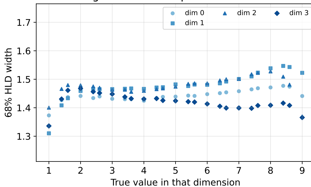
normal: HLD width per dimension
