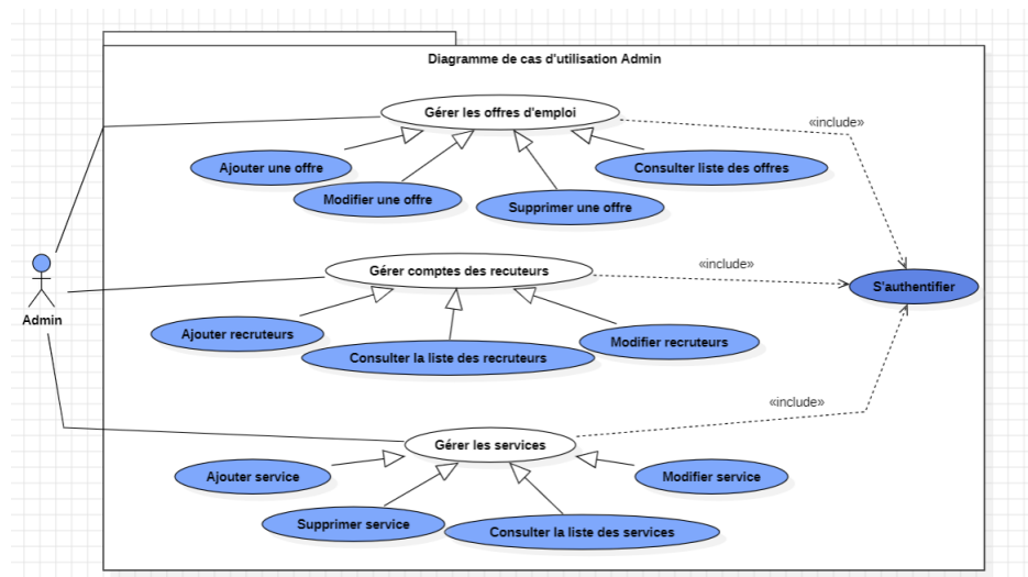
FIGURE 11 – Diagramme de cas d'utilisation de l'administrateur
