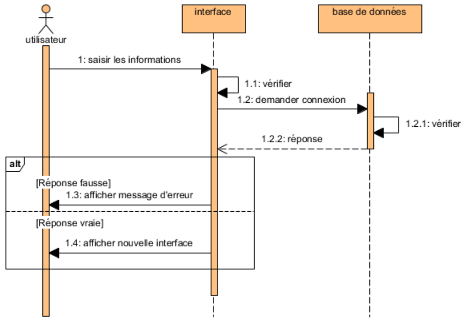
FIGURE 14 – Diagramme de séquence du mécanisme d'authentification
