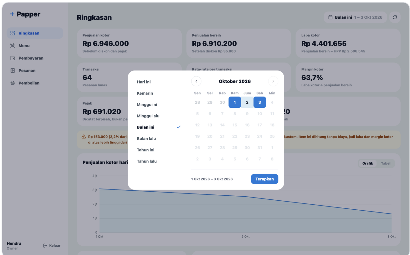
O-02 · Pemilih periode dengan pintasan dan kalender
