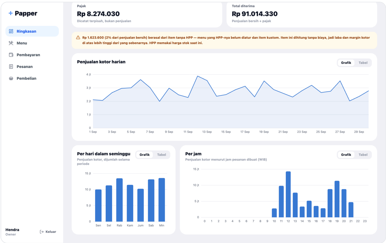
O-03 · Ringkasan: grafik harian, per hari dalam seminggu, dan per jam
