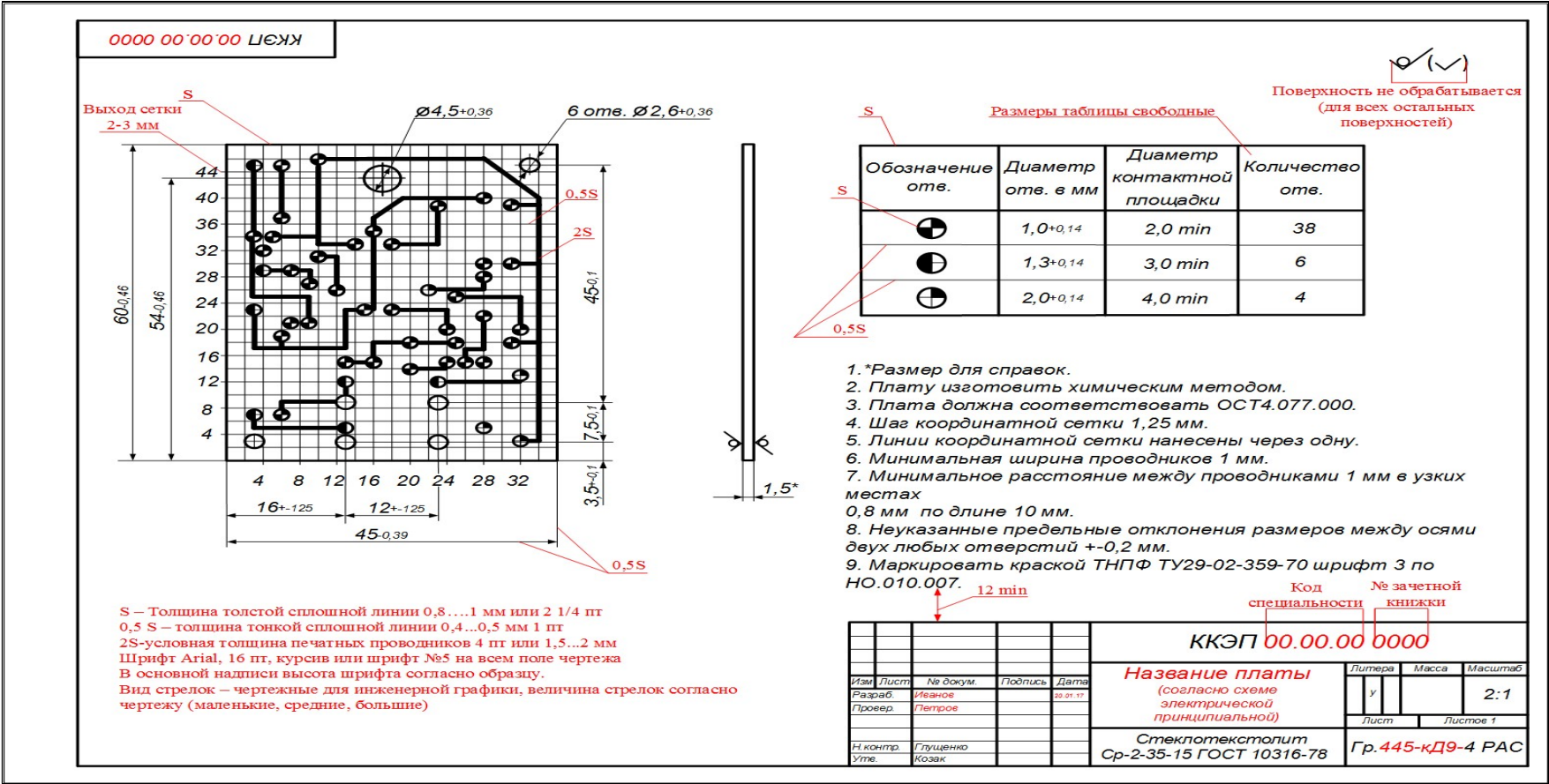
Рисунок Р.1 Схема платы
