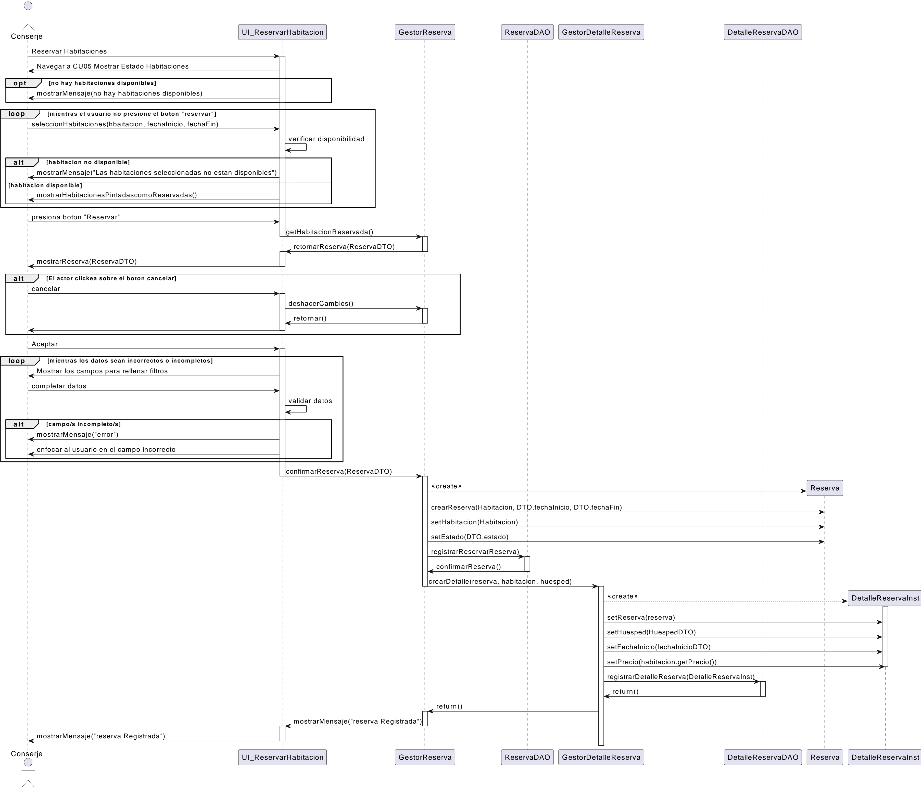
Diagrama_Secuencia_ CU04
