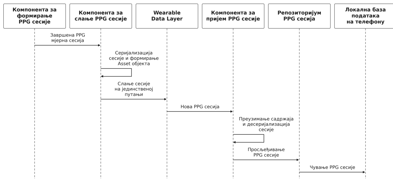
Слика 11: Ток преноса и чувања PPG мјерне сесије.
