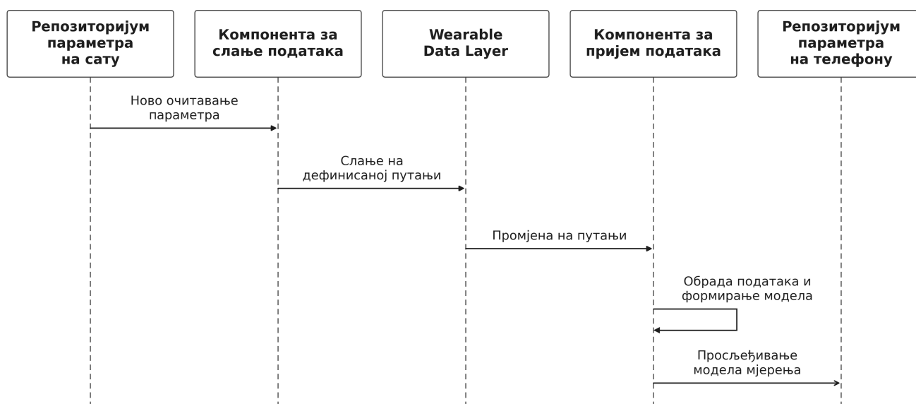
Слика 10: Ток преноса тренутних физиолошких вриједности.
