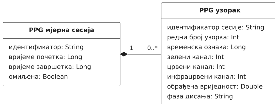
Слика 12: Дијаграм класа модела PPG мјерне сесије.
