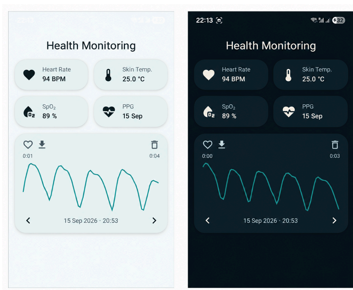
Слика 13: Главни екран мобилне апликације у свијетлој и тамној теми.
