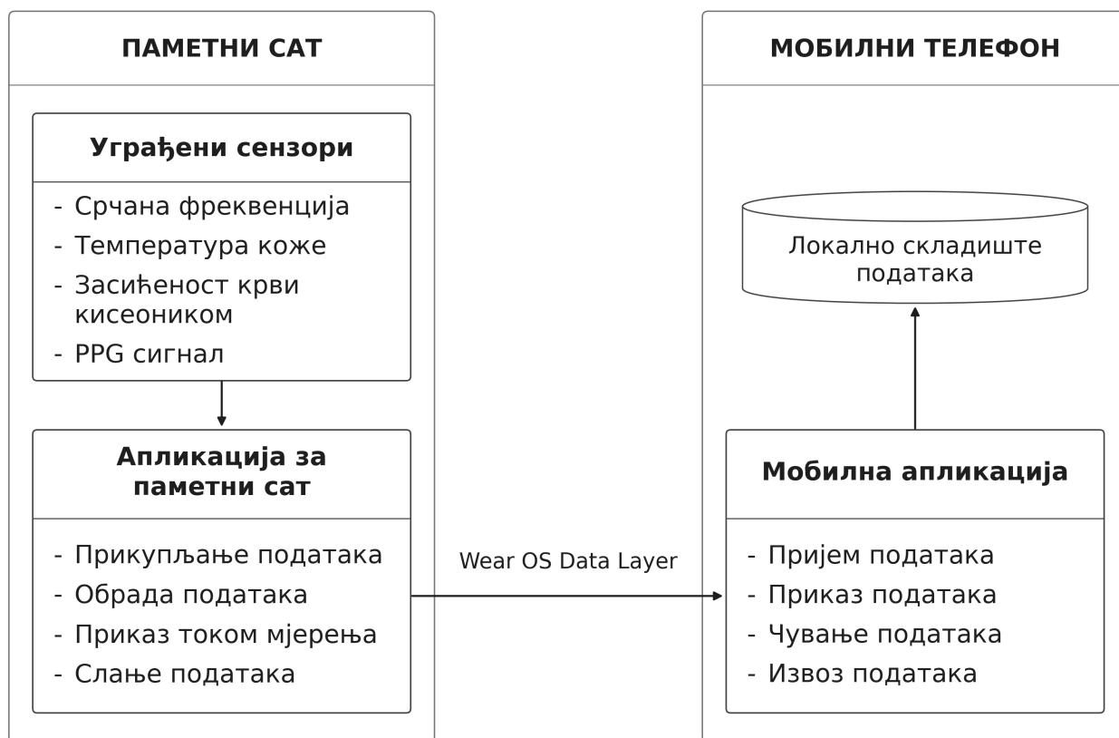
Слика 4: Архитектура система.
