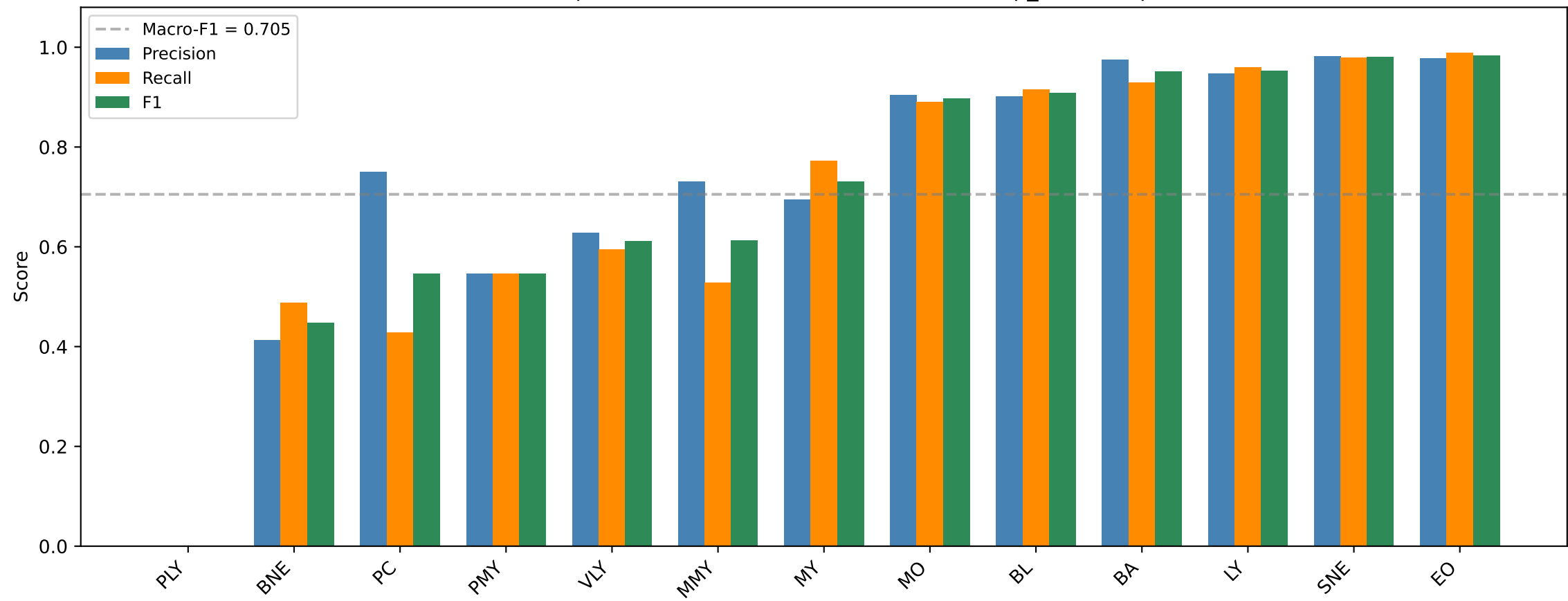
Per-class precision / recall / F1 on validation (deep_9 no-morph)
