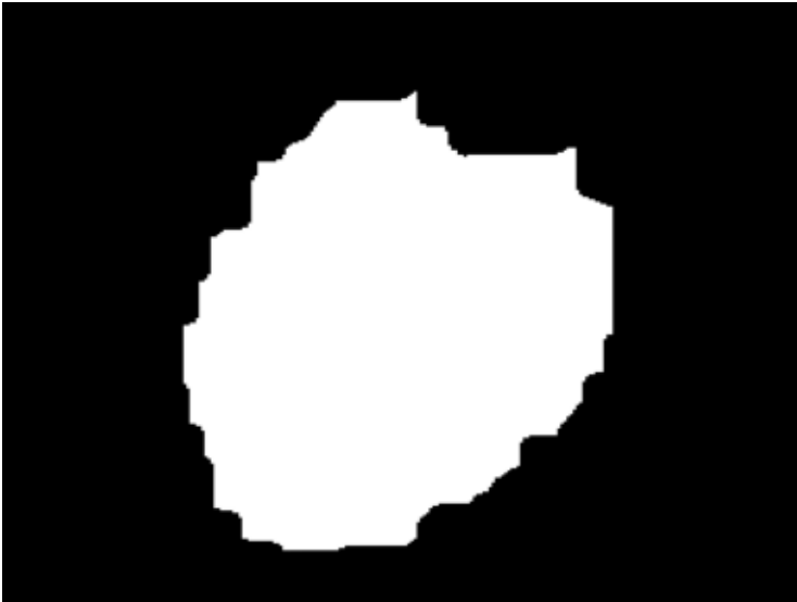
SRM Dice 0.943
