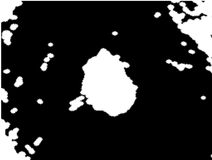
LBP Dice 0.576
