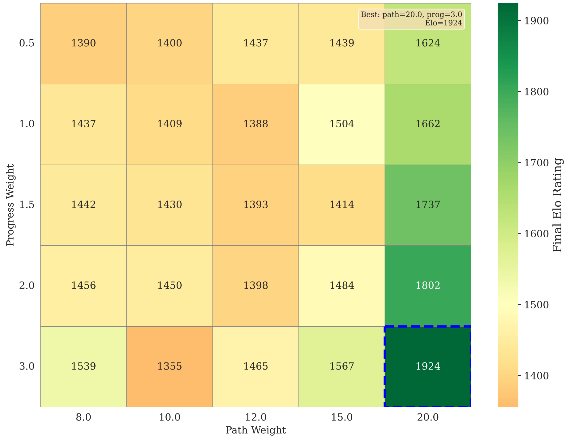
Hyperparameter Performance (Wall Weight = 2.0)
