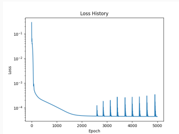
Rysunek 5: Historia funkcji kosztu (skala logarytmiczna).
