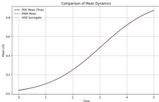
Rysunek 7: Porównanie średniej przestrzennej u(t) dla trzech modeli.
