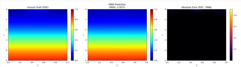
Rysunek 6: Porównanie rozwiązania referencyjnego (PDE), predykcji PINN oraz błędu absolutnego.
