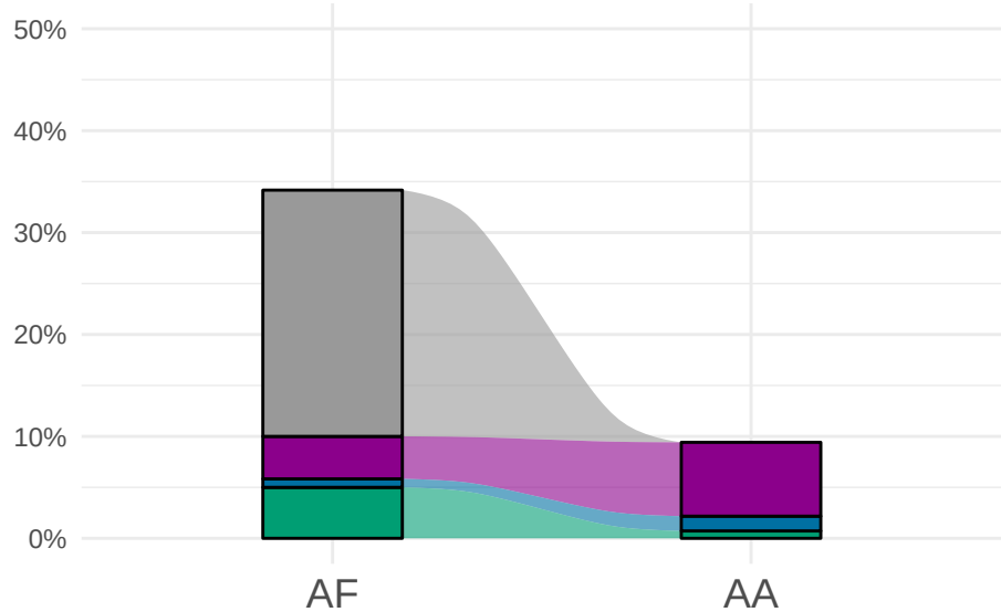
Bolitophagus reticulatus
