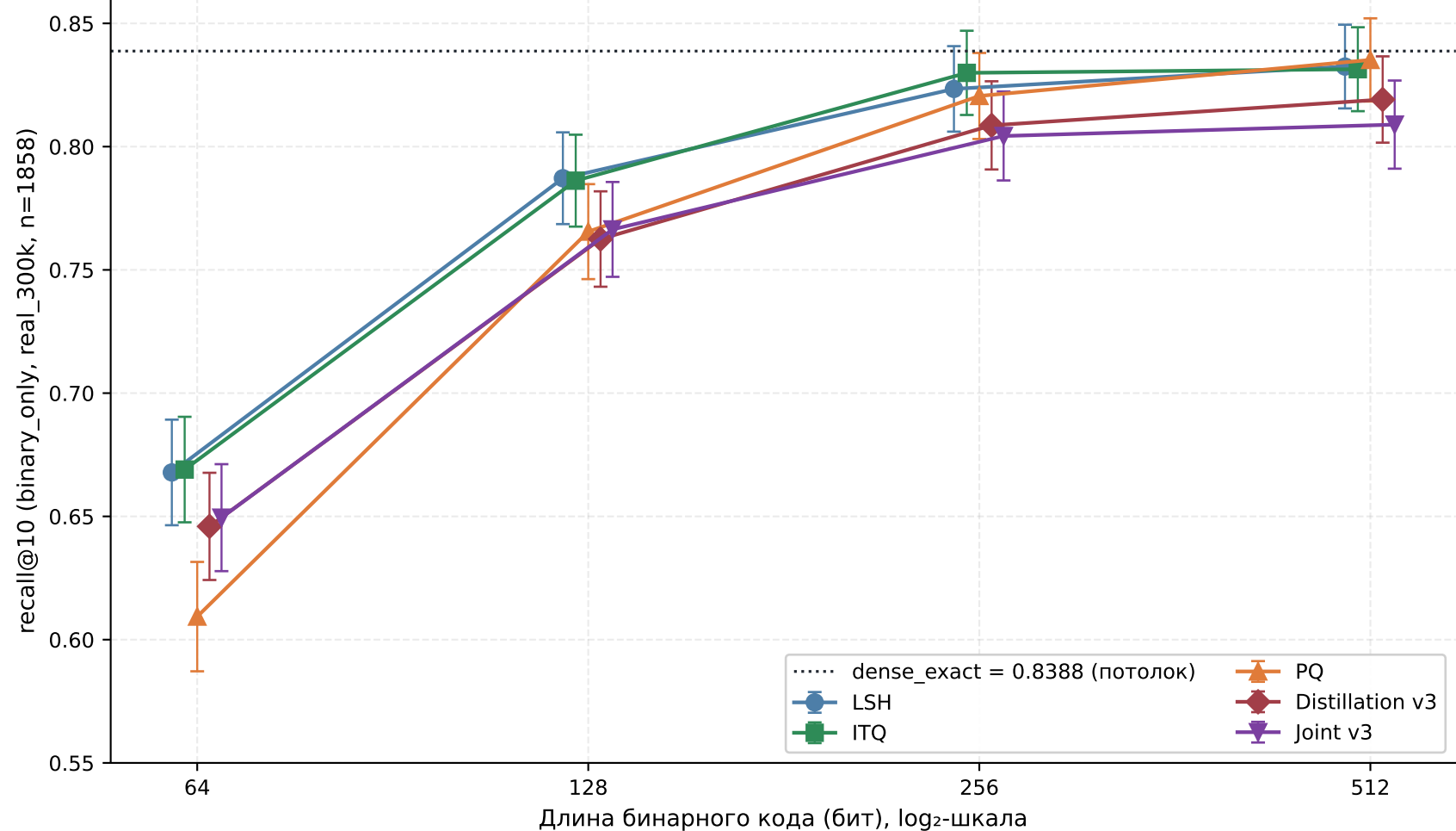
Рис. 5.3. Зависимость recall@10 от длины кода в режиме binary_only на real_300k
