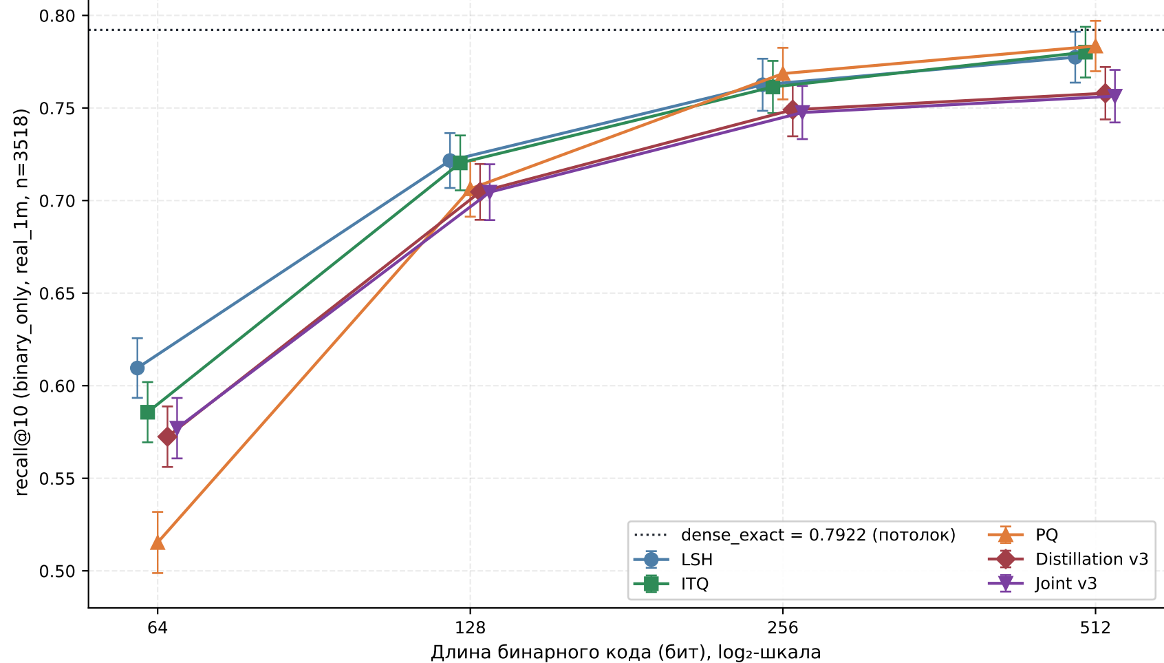
Рис. 5.4. Зависимость recall@10 от длины кода в режиме binary_only на real_1m
