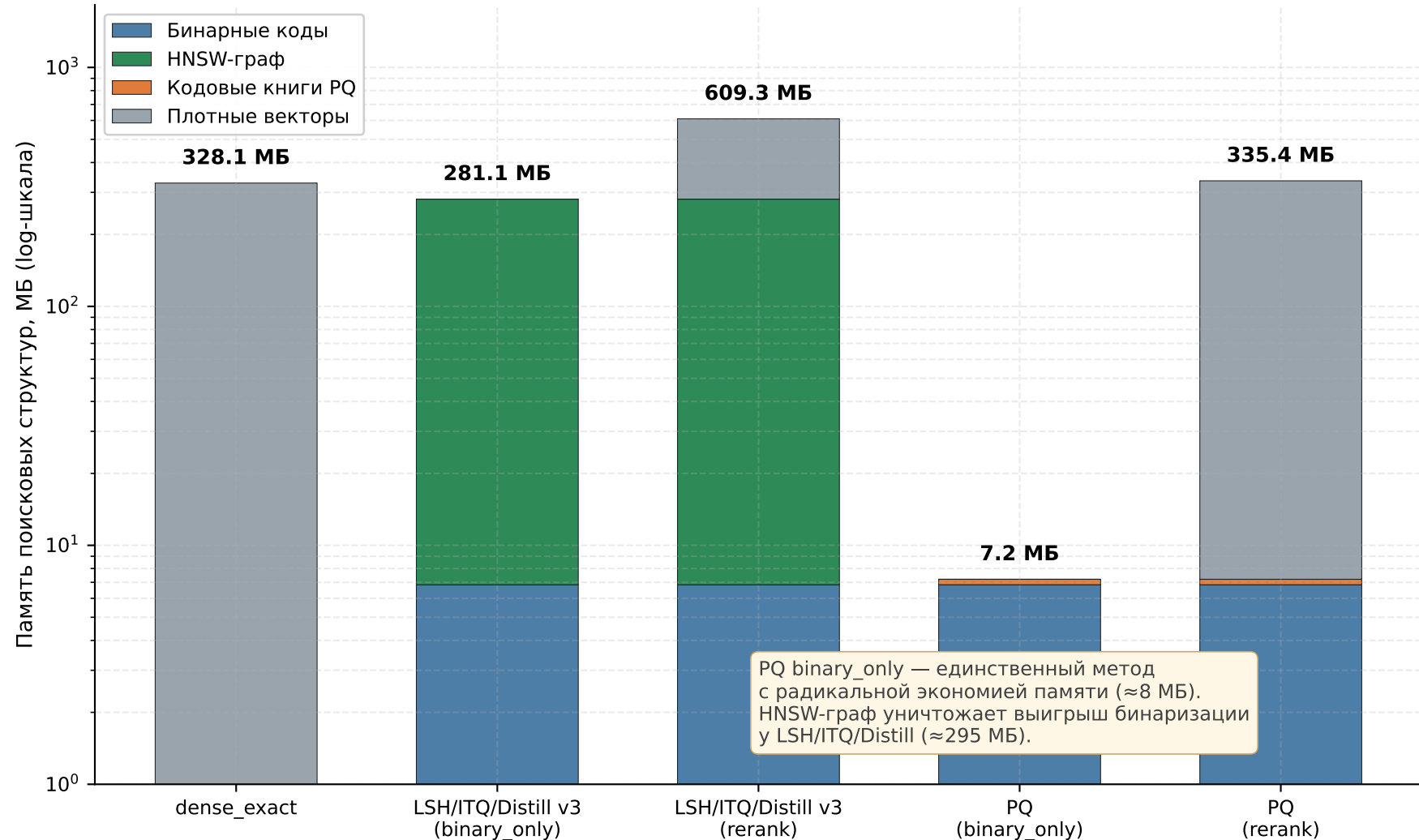
Рис. 5.5. Совокупная память поисковых структур по компонентам (256 бит, real_300k = 224 017 документов)
