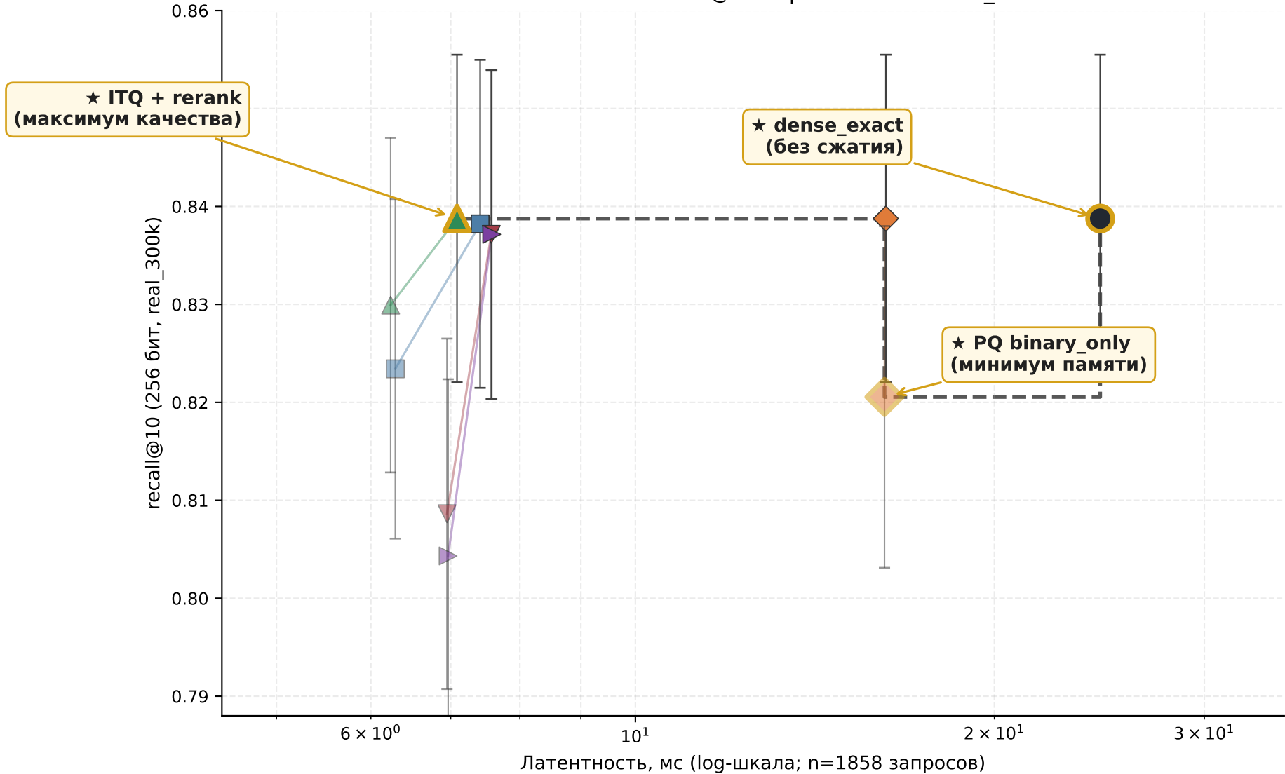
Рис. 5.7. Pareto-frontier «латентность × recall@10» при 256 бит на real_300k
