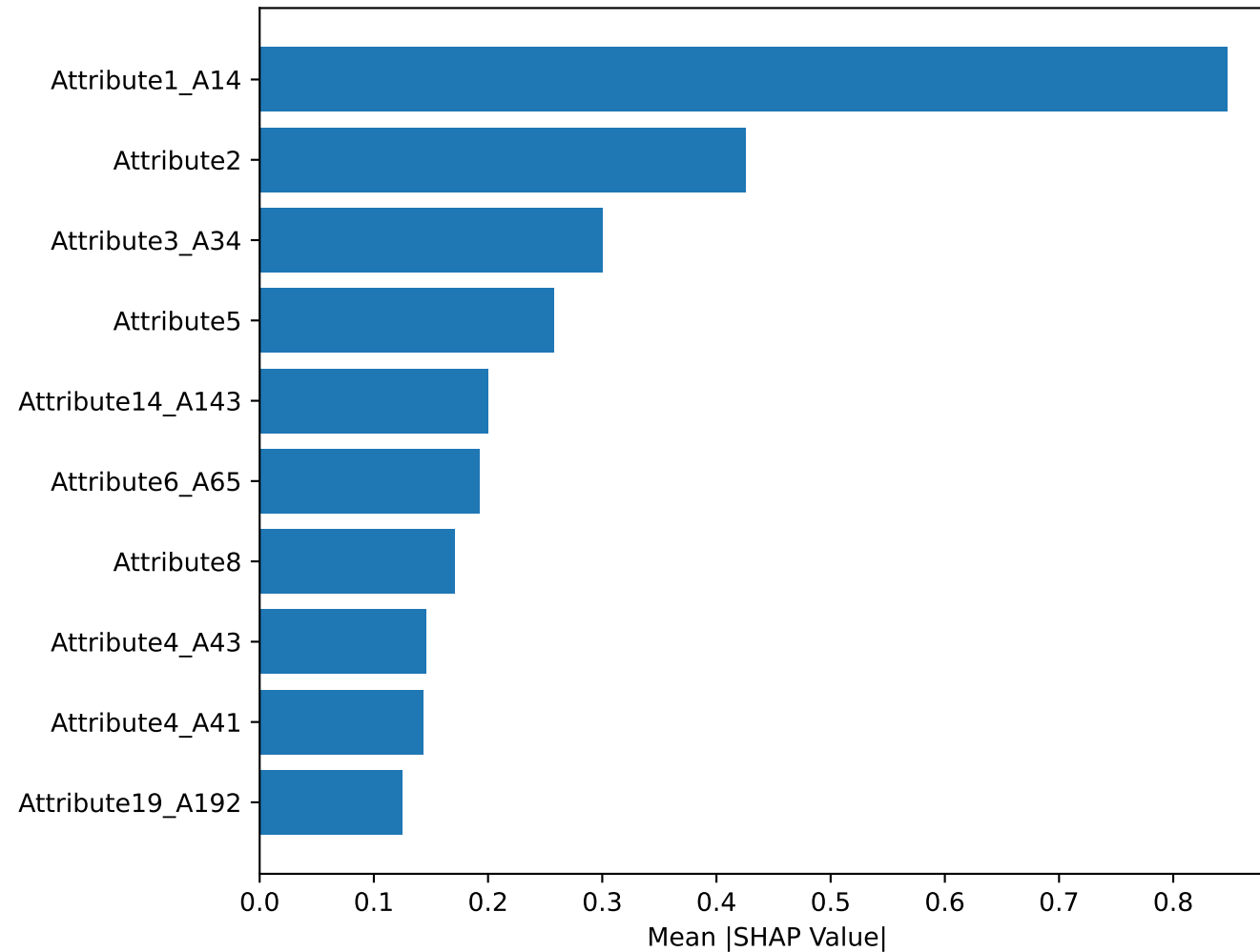
SHAP Top 10 — XGBoost
