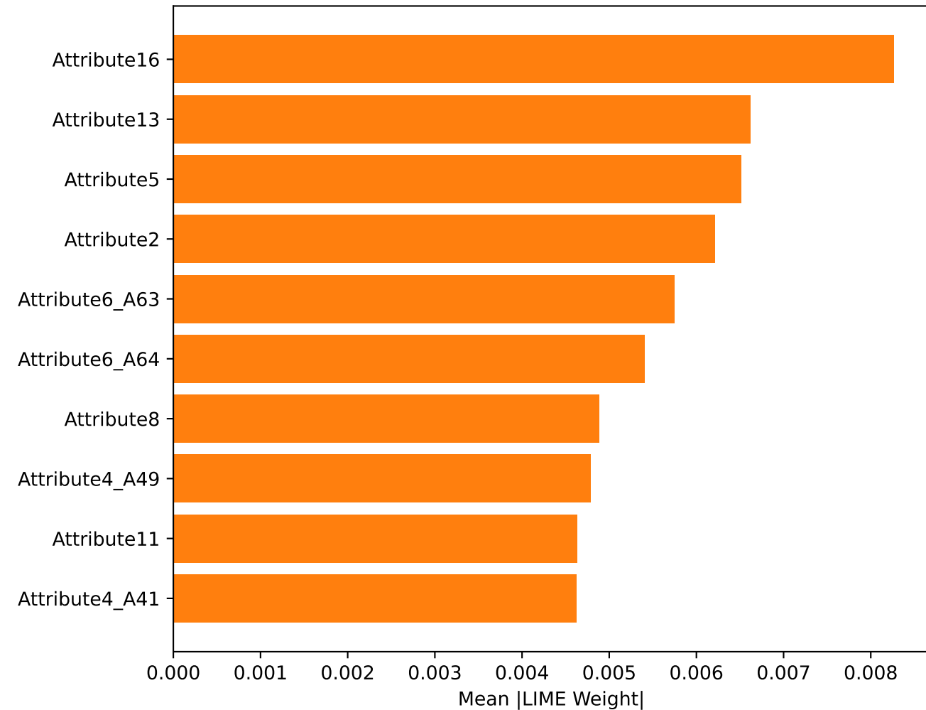
LIME Top 10 — XGBoost
