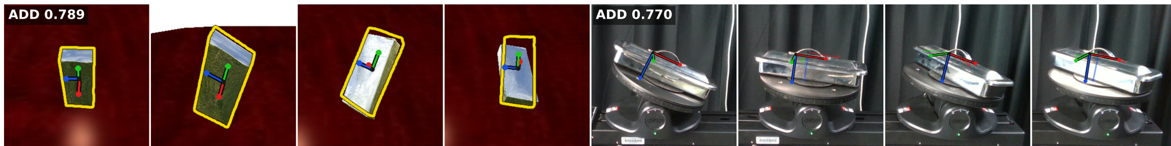
Ours
