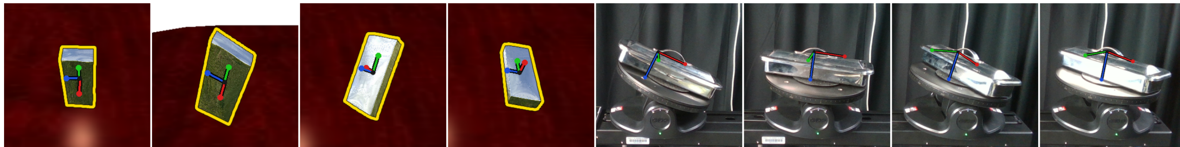
ADD 0.033
