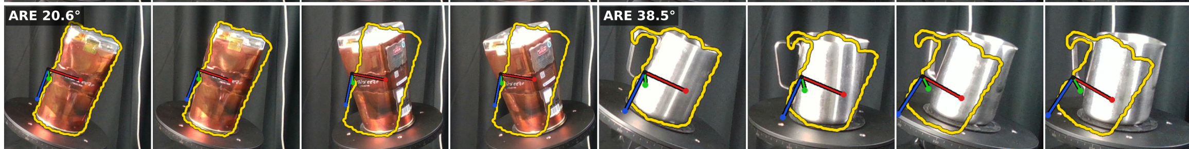
LoFTR
