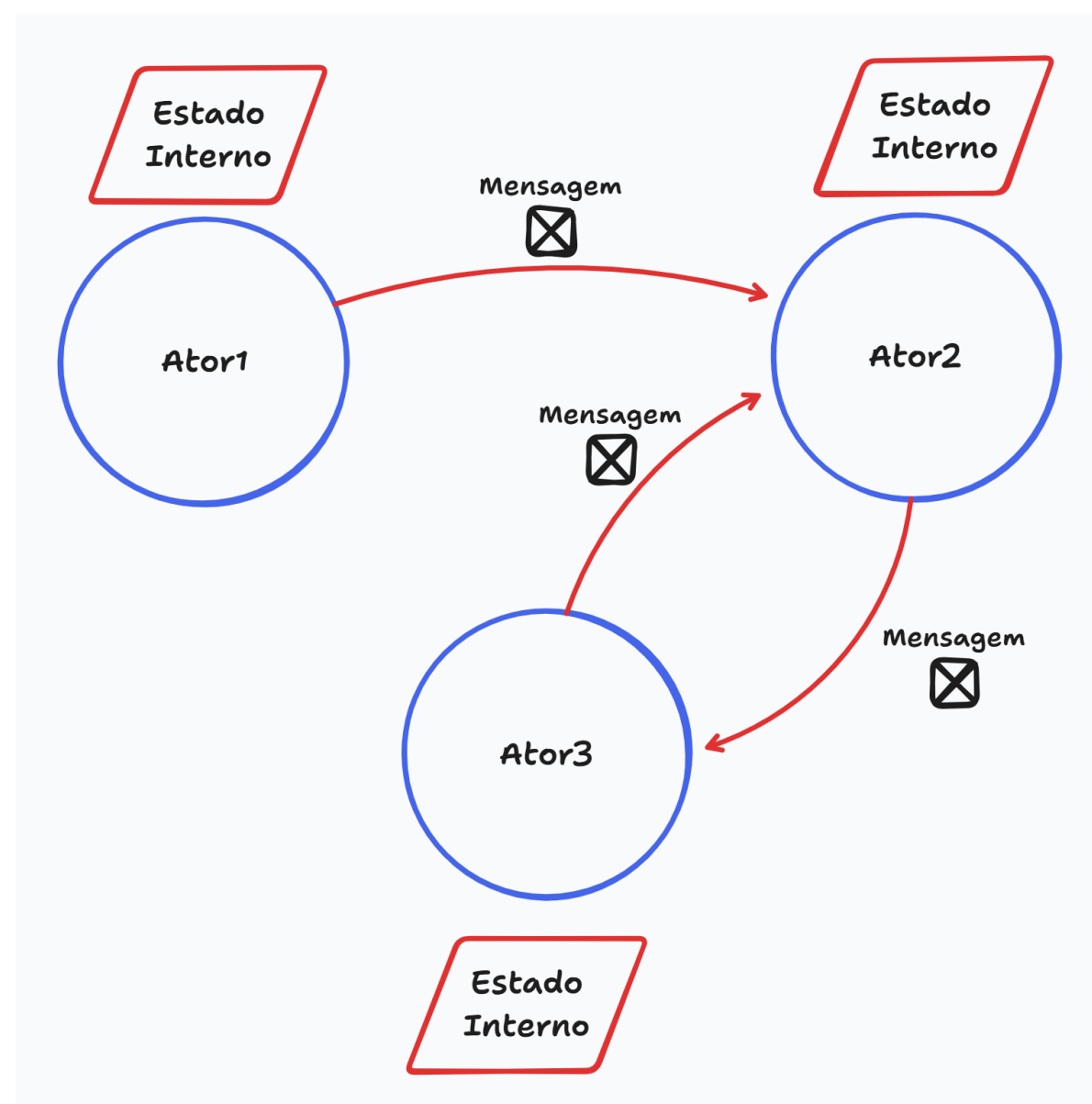
Figure 1: Comunicação entre atores
