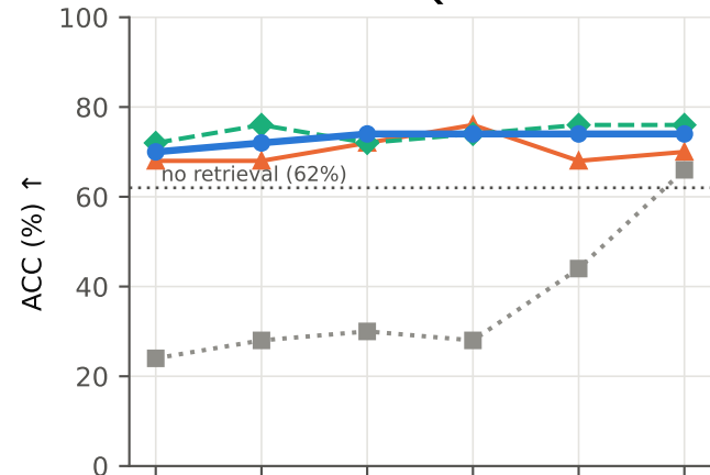
NQ
