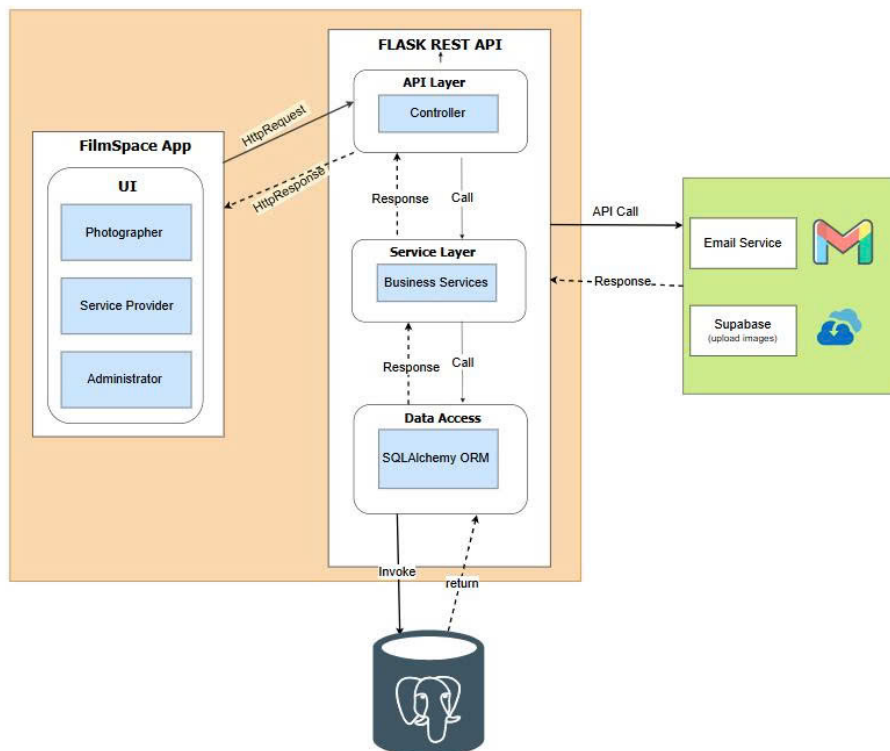
Figure IV.1: Kiến trúc tổng thể của hệ thống
