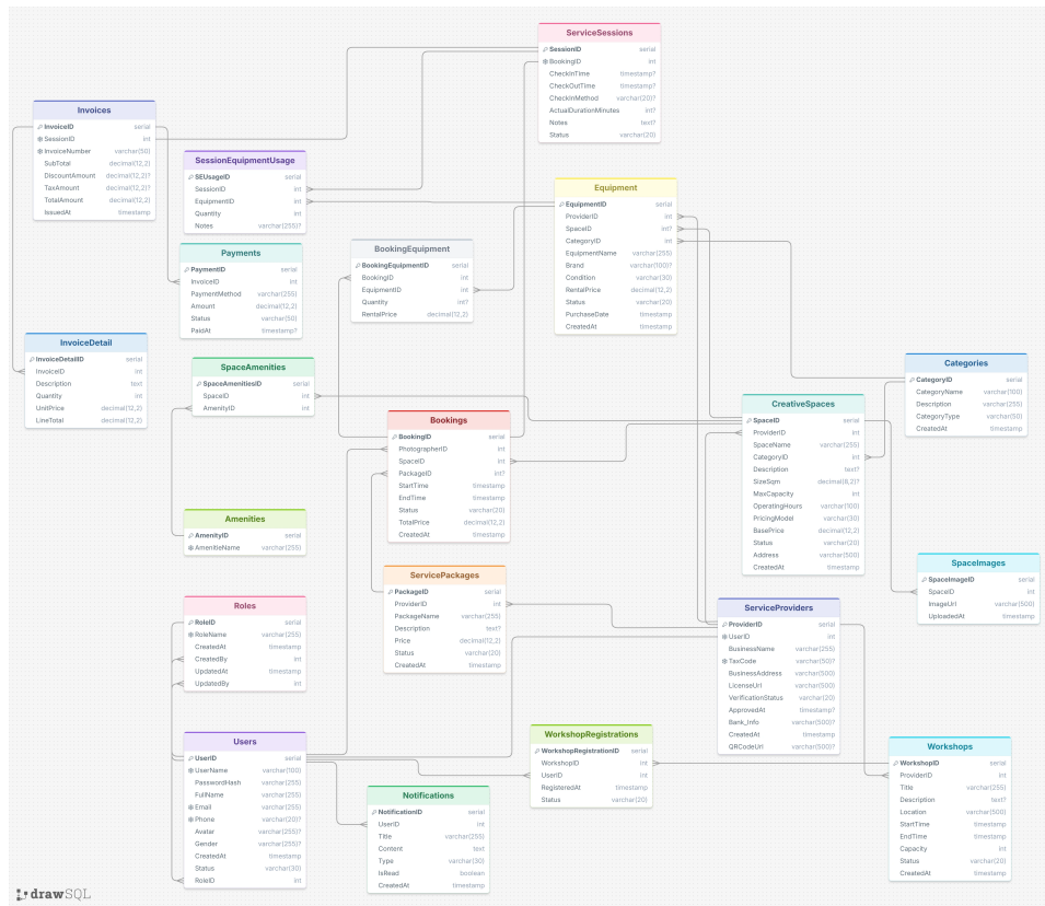
Figure III.6: Sơ đồ quan hệ thực thể của hệ thống
