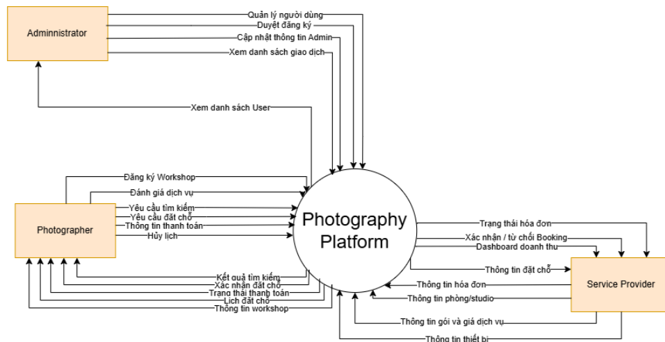
Figure III.1: Sơ đồ ngữ cảnh của hệ thống
