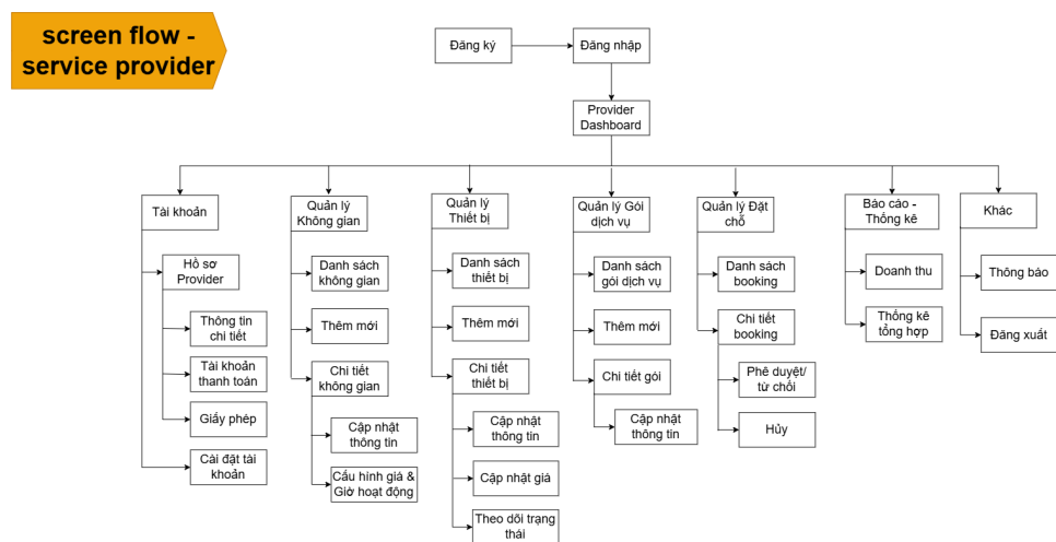
Figure III.4: Screen Flow của Service Provider
