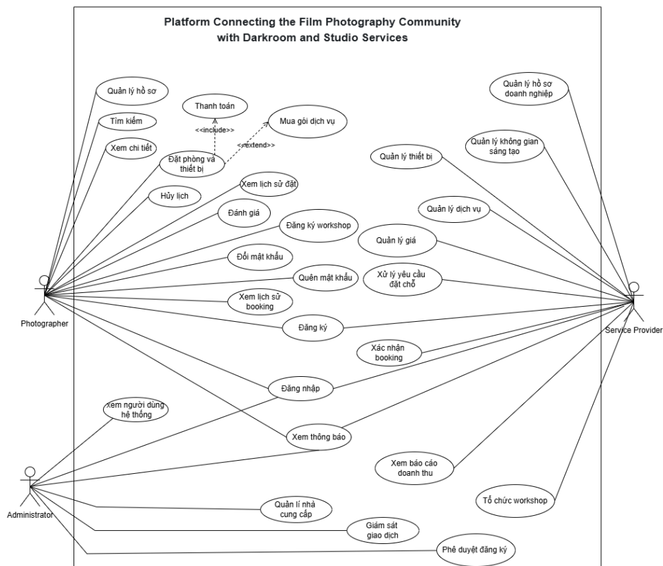
Figure III.2: Sơ đồ Use Case của hệ thống
