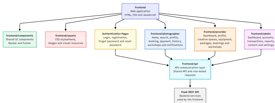
Figure IV.2: Kiến trúc Frontend
