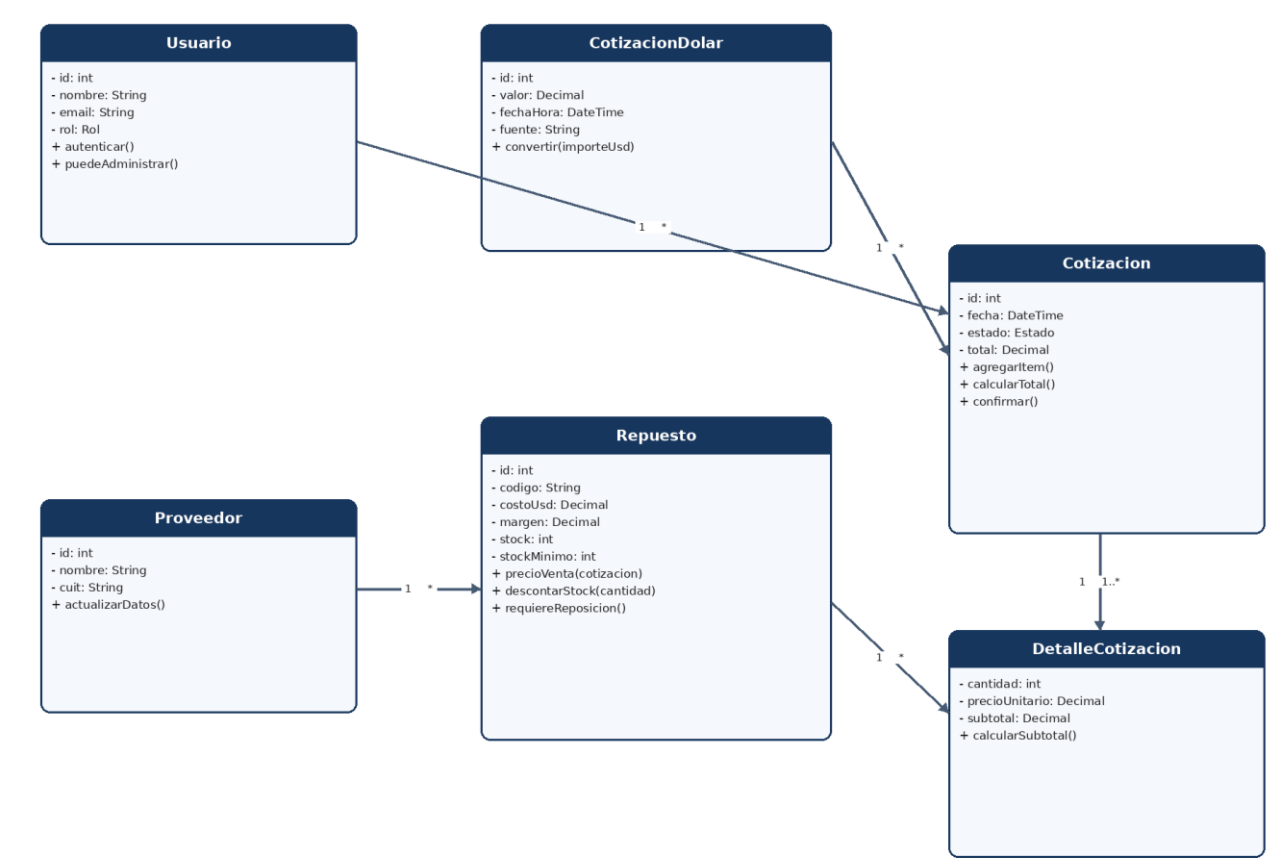
Figura 4. Diagrama de clases UML de StockPar
