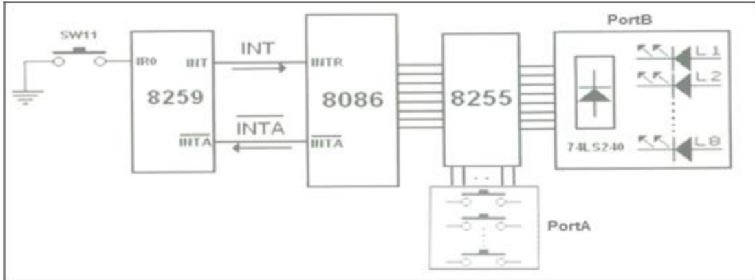
Donanımsal Blok Şema
