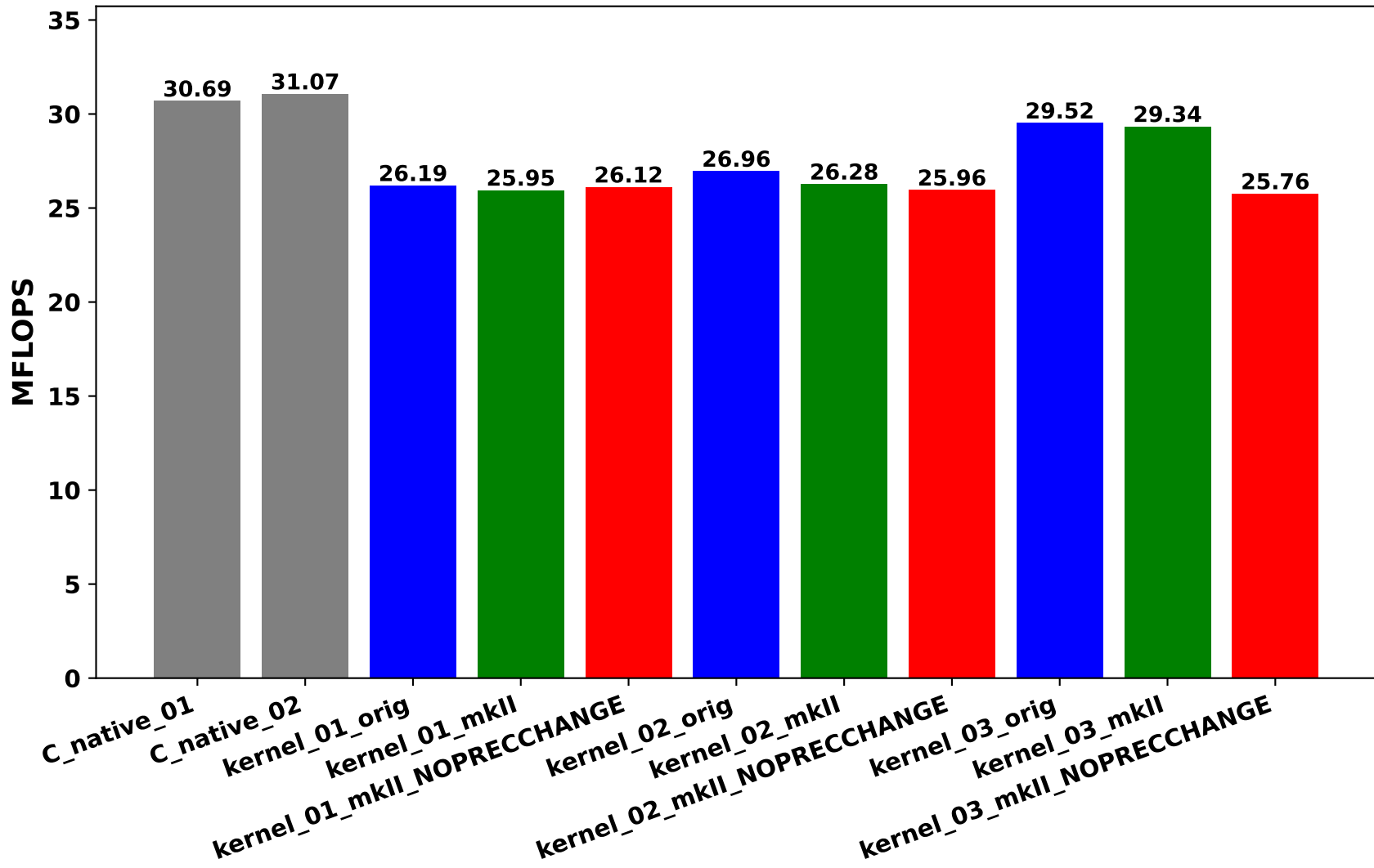
Rgemm serial benchmark on Ryzen 3970X 32-Core (prec=512)
