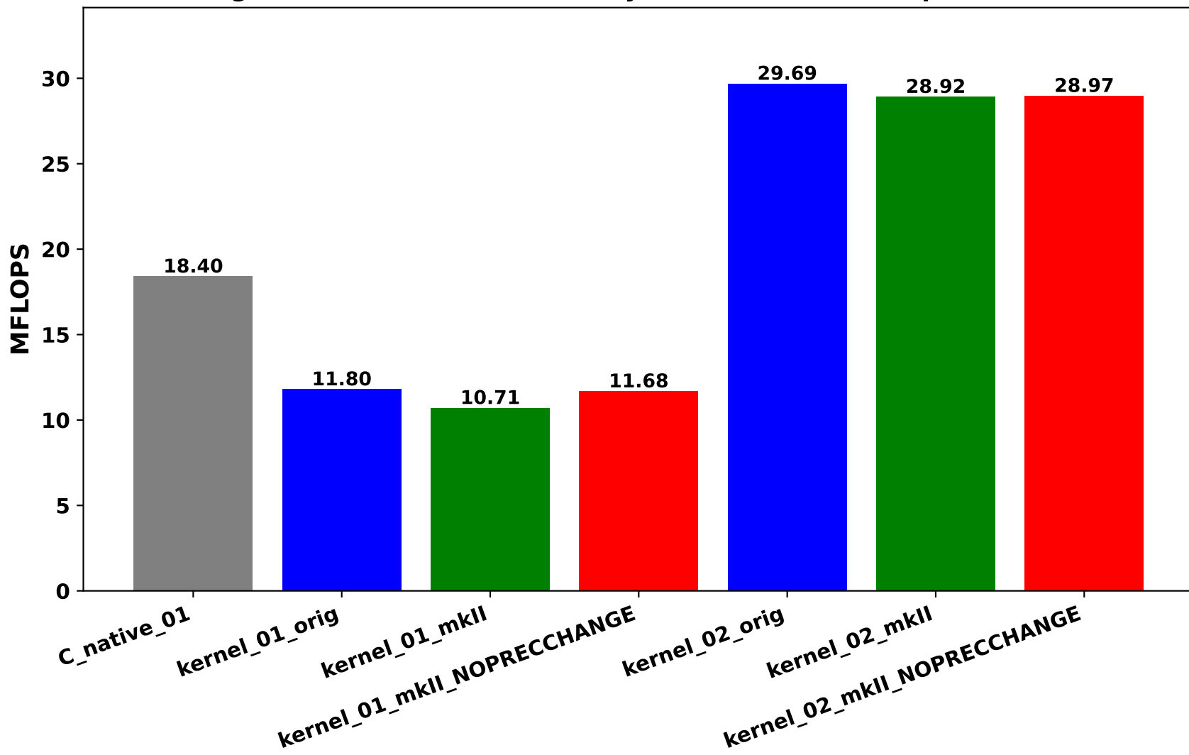
Rgemv serial benchmark on Ryzen 3970X 32-Core (prec=512)
