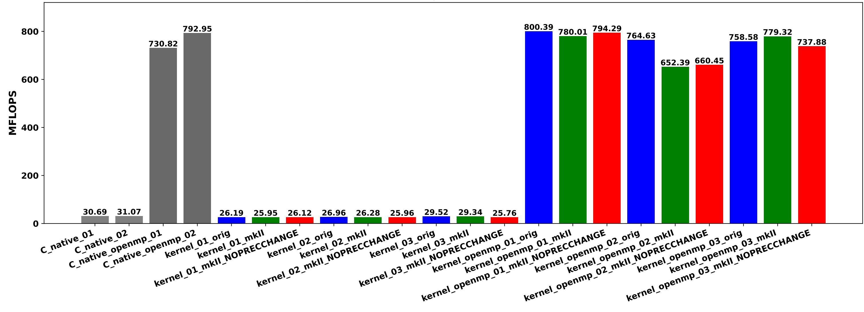
Rgemm benchmark on Ryzen 3970X 32-Core (prec=512)
